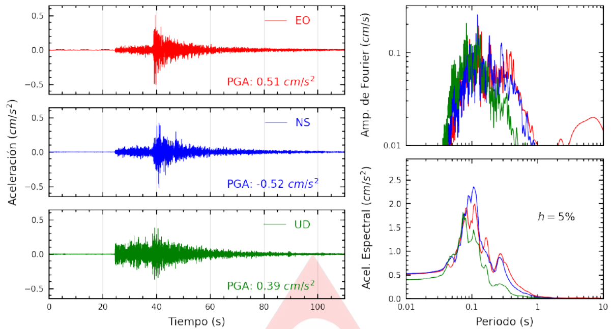
Figura A.1: Registros tiempo-historia, espectros de Fourier y de respuesta en las direcciones EO, NS y UD de la estación SCPIU. Sismo de Mancora, Talara - Piura de 2025-02-27, 03:05:25 (Hora local)
