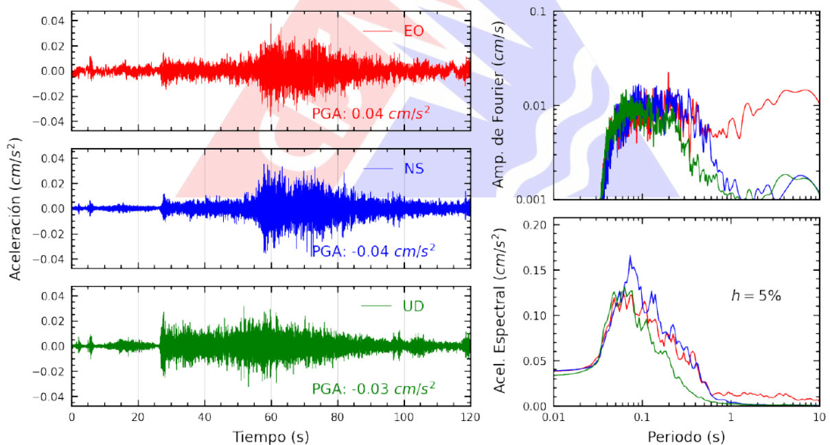
Figura A.2: Registros tiempo-historia, espectros de Fourier y de respuesta en las direcciones EO, NS y UD de la estación SCCHI. Sismo de Mancora, Talara - Piura de 2025-02-27, 03:05:25 (Hora local)
