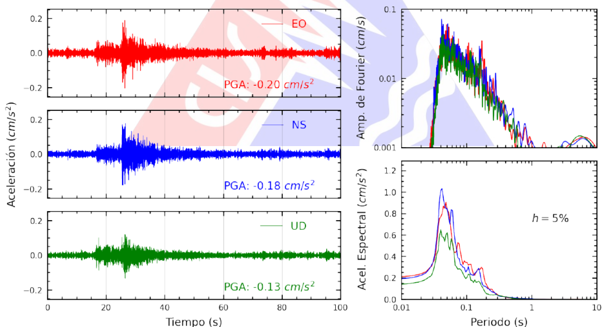
Figura A.2: Registros tiempo-historia, espectros de Fourier y de respuesta en las direcciones EO, NS y UD de la estación BORJA. Sismo de Chilca, Cañete - Lima de 2025-03-02, 07:36:43 (Hora local)
