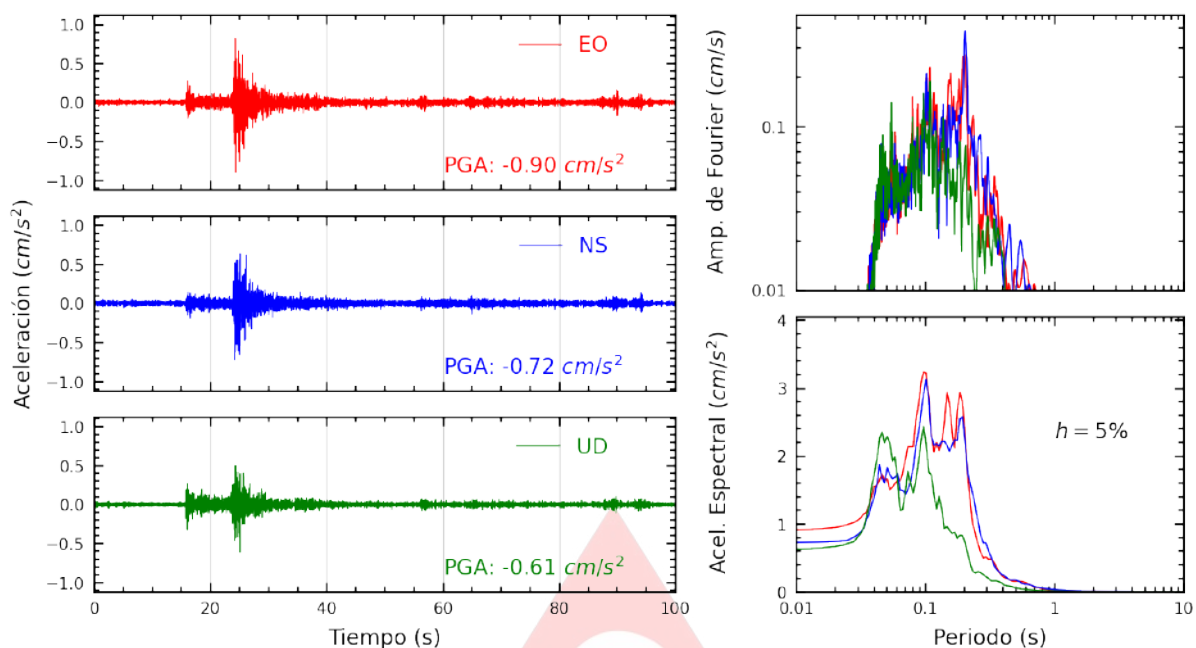
Figura A.1: Registros tiempo-historia, espectros de Fourier y de respuesta en las direcciones EO, NS y UD de la estación SCCHO. Sismo de Chilca, Cañete - Lima de 2025-03-02, 07:36:43 (Hora local)
