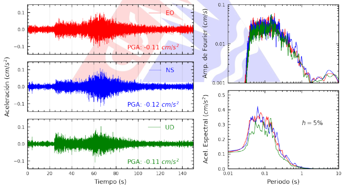
Figura A.2: Registros tiempo-historia, espectros de Fourier y de respuesta en las direcciones EO, NS y UD de la estación BORJA. Sismo de Ica, Ica - Ica de 2025-03-02, 06:02:04 (Hora local)
