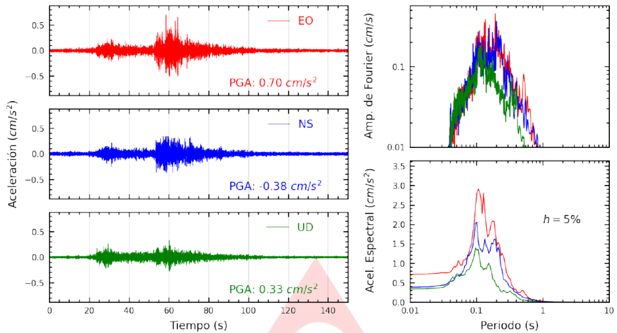
Figura A.1: Registros tiempo-historia, espectros de Fourier y de respuesta en las direcciones EO, NS y UD de la estación SCCHO. Sismo de Ica, Ica - Ica de 2025-03-02, 06:02:04 (Hora local)
