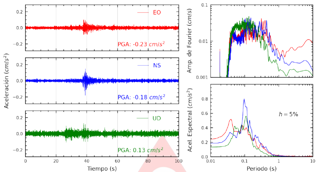
Figura A.1: Registros tiempo-historia, espectros de Fourier y de respuesta en las direcciones EO, NS y UD de la estación SCPIU. Sismo de Talara, Talara - Piura de 2025-03-03, 13:11:08 (Hora local)
