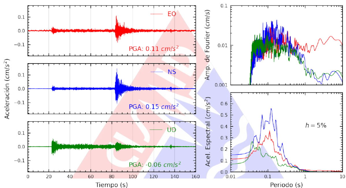
Figura A.3: Registros tiempo-historia, espectros de Fourier y de respuesta en las direcciones EO, NS y UD de la estación SCCHI. Sismo de Pucallpa, Coronel Portillo - Ucayali de 2025-03-05, 02:36:38 (Hora local)
