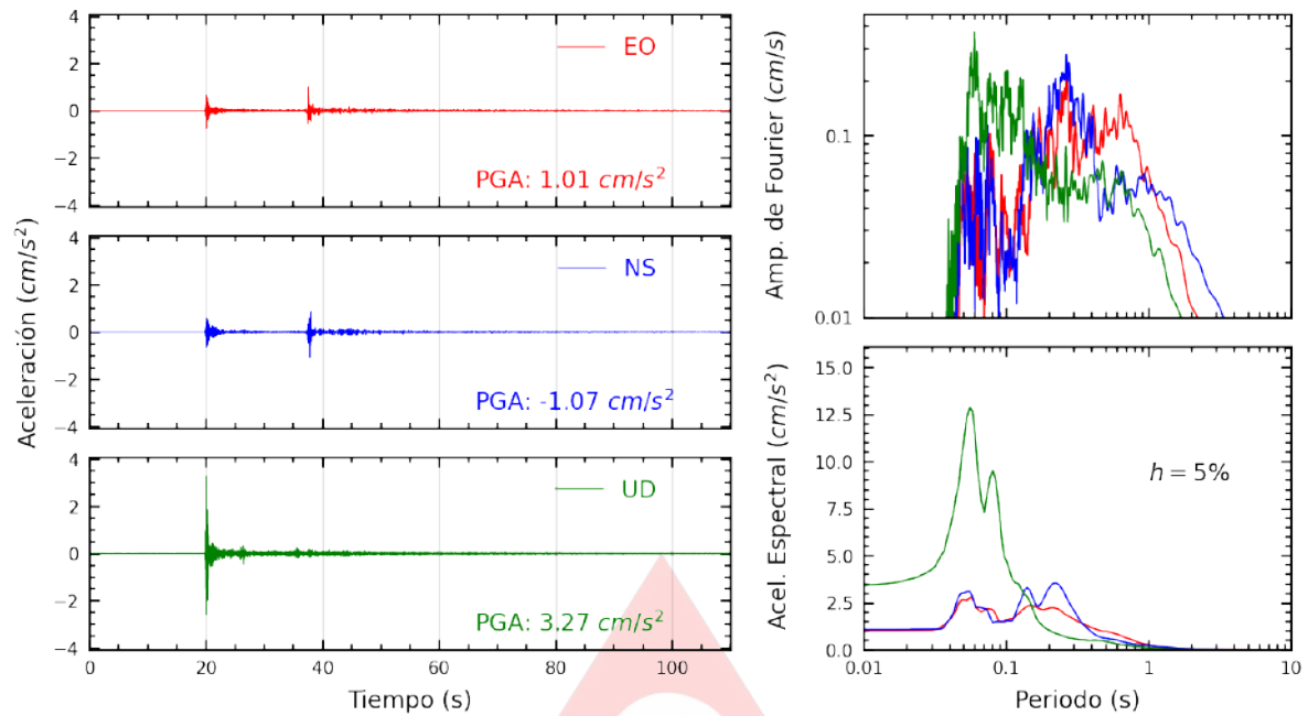
Figura A.1: Registros tiempo-historia, espectros de Fourier y de respuesta en las direcciones EO, NS y UD de la estación SCPUC. Sismo de Pucallpa, Coronel Portillo - Ucayali de 2025-03-05, 02:36:38 (Hora local)
