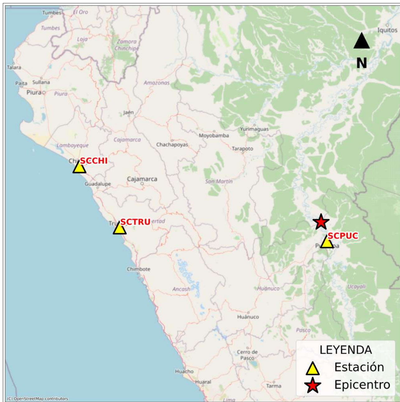
Figura 2: Mapa de ubicación de la(s) estación(es) acelerográfica(s) que registraron el Sismo de Pucallpa, Coronel Portillo - Ucayali del 05 de marzo de 2025 a las 02:36:38 (hora local)
