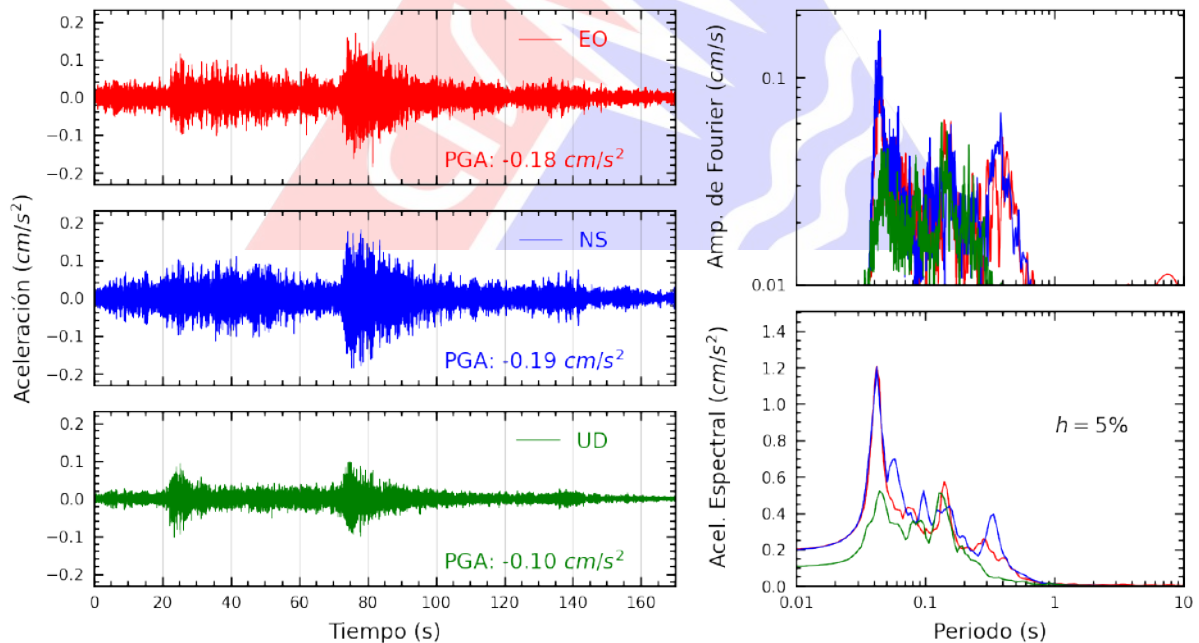
Figura A.2: Registros tiempo-historia, espectros de Fourier y de respuesta en las direcciones EO, NS y UD de la estación SCTRU. Sismo de Pucallpa, Coronel Portillo - Ucayali de 2025-03-05, 02:36:38 (Hora local)
