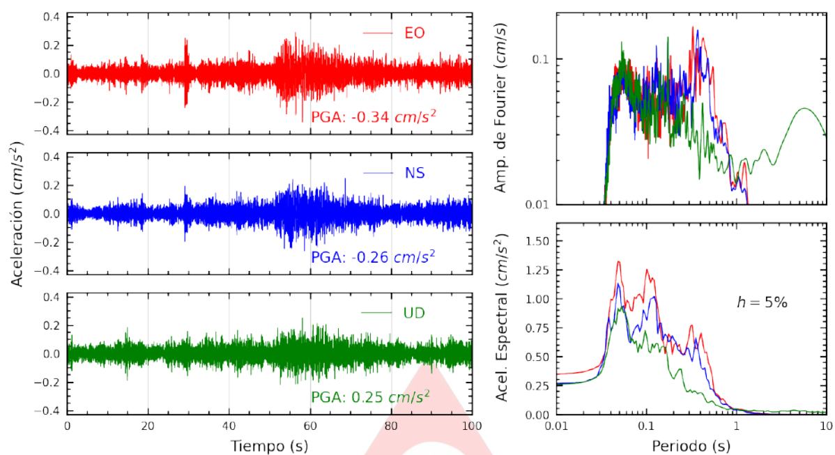
Figura A.1: Registros tiempo-historia, espectros de Fourier y de respuesta en las direcciones EO, NS y UD de la estación SCARQ. Sismo de Ilo, Ilo - Moquegua de 2025-03-06, 13:13:35 (Hora local)
