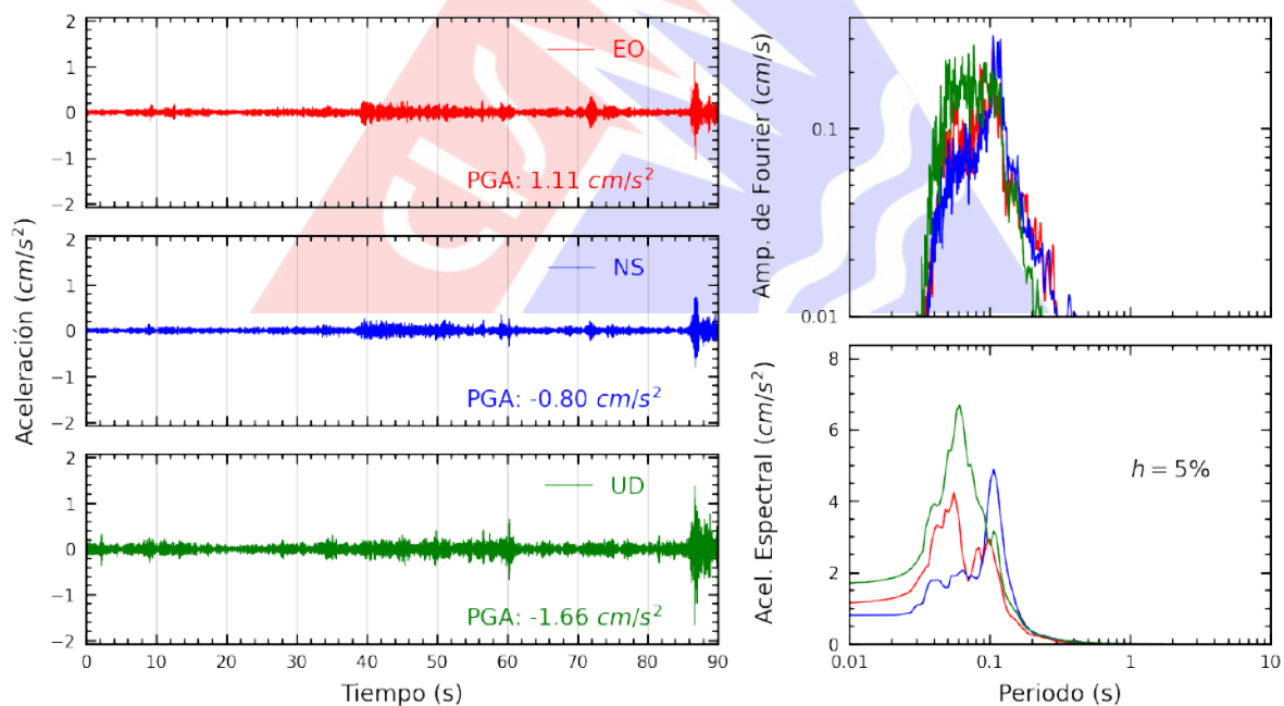
Figura A.2: Registros tiempo-historia, espectros de Fourier y de respuesta en las direcciones EO, NS y UD de la estación SCOLI. Sismo de Mala, Cañete - Lima de 2025-03-07, 22:47:44 (Hora local)
