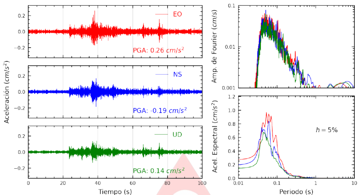
Figura A.1: Registros tiempo-historia, espectros de Fourier y de respuesta en las direcciones EO, NS y UD de la estación BORJA. Sismo de Mala, Cañete - Lima de 2025-03-07, 22:47:44 (Hora local)
