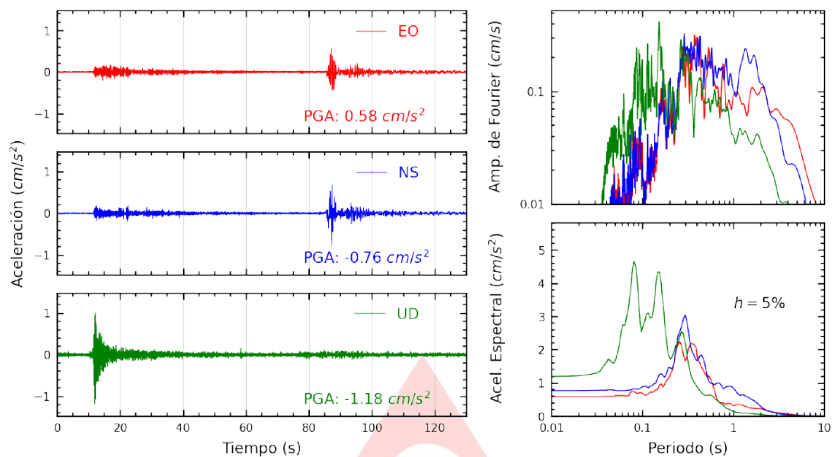
Figura A.1: Registros tiempo-historia, espectros de Fourier y de respuesta en las direcciones EO, NS y UD de la estación SCPUC. Sismo de Esperanza, Purus - Ucayali de 2025-03-11, 09:07:55 (Hora local)
