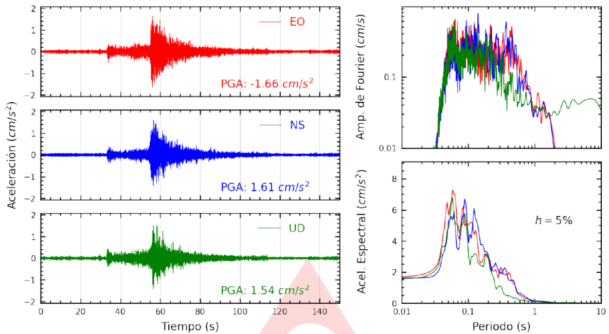
Figura A.1: Registros tiempo-historia, espectros de Fourier y de respuesta en las direcciones EO, NS y UD de la estación SCARQ. Sismo de Caraveli, Caraveli - Arequipa de 2025-03-15, 21:20:53 (Hora local)
