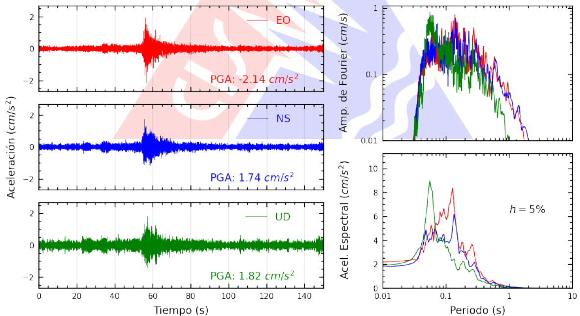
Figura A.2: Registros tiempo-historia, espectros de Fourier y de respuesta en las direcciones EO, NS y UD de la estación SCAR2. Sismo de Caraveli, Caraveli - Arequipa de 2025-03-15, 21:20:53 (Hora local)
