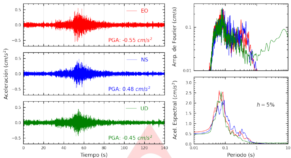
Figura A.1: Registros tiempo-historia, espectros de Fourier y de respuesta en las direcciones EO, NS y UD de la estación SCARQ. Sismo de Ocoña, Camana - Arequipa de 2025-03-17, 18:05:13 (Hora local)
