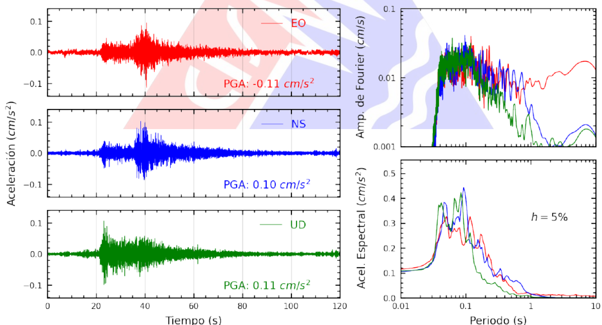
Figura A.2: Registros tiempo-historia, espectros de Fourier y de respuesta en las direcciones EO, NS y UD de la estación SCCHI. Sismo de Olmos, Lambayeque - Lambayeque de 2025-03-17, 11:25:11 (Hora local)
