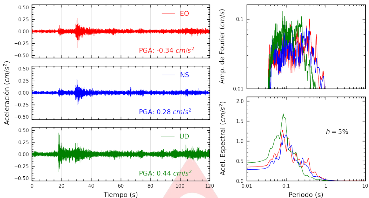
Figura A.1: Registros tiempo-historia, espectros de Fourier y de respuesta en las direcciones EO, NS y UD de la estación SCPIU. Sismo de Olmos, Lambayeque - Lambayeque de 2025-03-17, 11:25:11 (Hora local)
