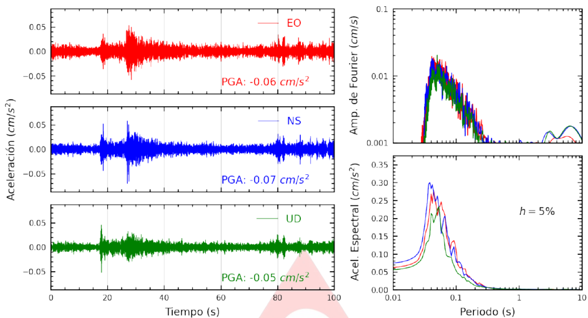
Figura A.1: Registros tiempo-historia, espectros de Fourier y de respuesta en las direcciones EO, NS y UD de la estación BORJA. Sismo de Ancon, Lima - Lima de 2025-03-19, 01:02:13 (Hora local)
