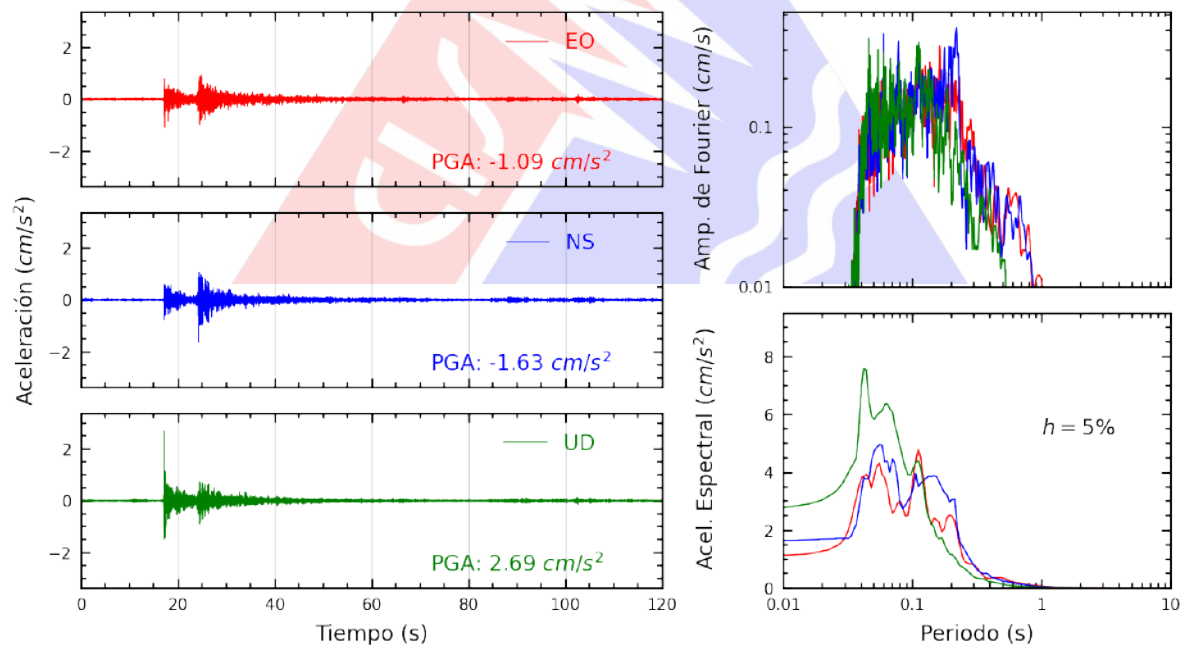
Figura A.2: Registros tiempo-historia, espectros de Fourier y de respuesta en las direcciones EO, NS y UD de la estación SCCHO. Sismo de Lima, Lima - Lima de 2025-03-22, 00:14:18 (Hora local)
