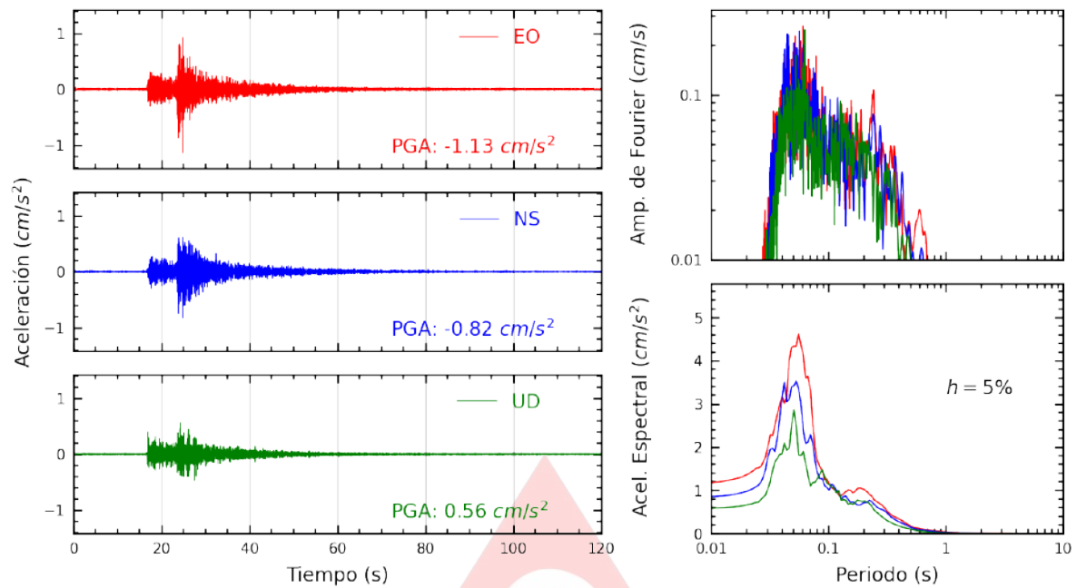
Figura A.1: Registros tiempo-historia, espectros de Fourier y de respuesta en las direcciones EO, NS y UD de la estación BORJA. Sismo de Lima, Lima - Lima de 2025-03-22, 00:14:18 (Hora local)
