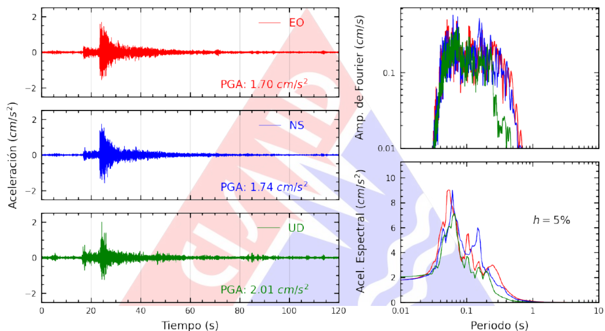
Figura A.3: Registros tiempo-historia, espectros de Fourier y de respuesta en las direcciones EO, NS y UD de la estación SCOLI. Sismo de Lima, Lima - Lima de 2025-03-22, 00:14:18 (Hora local)
