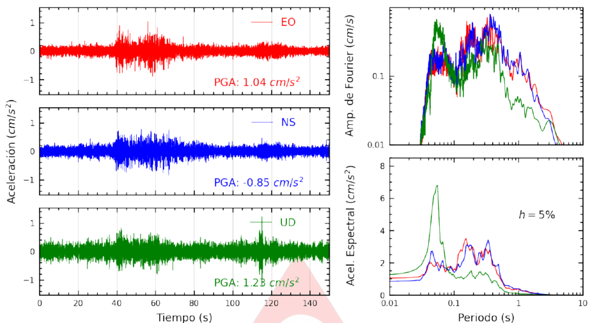
Figura A.1: Registros tiempo-historia, espectros de Fourier y de respuesta en las direcciones EO, NS y UD de la estación SCAR2. Sismo de Tacna, Tacna - Tacna de 2025-03-25, 17:55:51 (Hora local)
