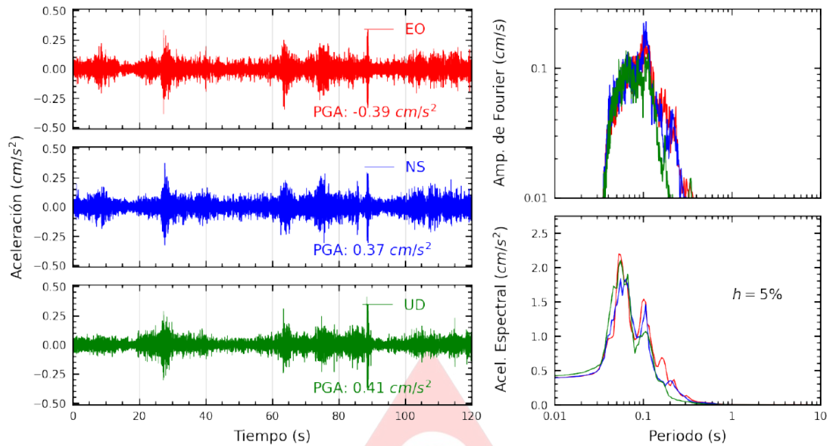
Figura A.1: Registros tiempo-historia, espectros de Fourier y de respuesta en las direcciones EO, NS y UD de la estación SCCHO. Sismo de Lima, Lima - Lima de 2025-03-28, 06:24:27 (Hora local)
