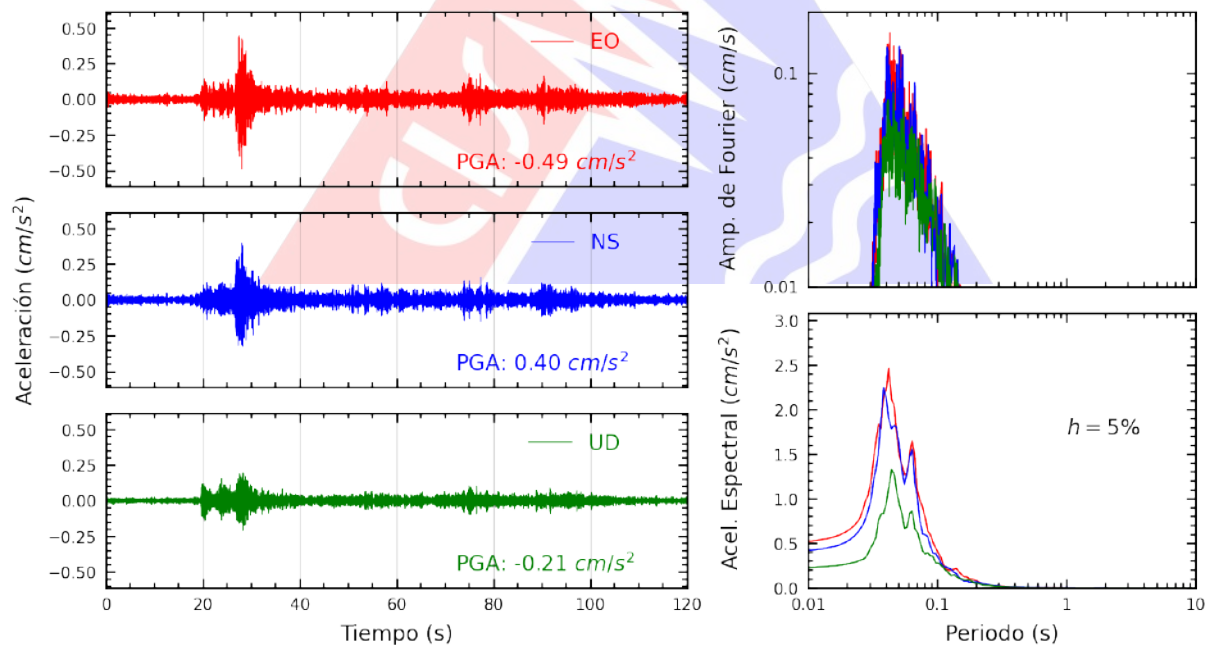
Figura A.2: Registros tiempo-historia, espectros de Fourier y de respuesta en las direcciones EO, NS y UD de la estación BORJA. Sismo de Lima, Lima - Lima de 2025-03-28, 06:24:27 (Hora local)
