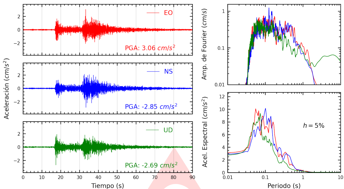
Figura A.1: Registros tiempo-historia, espectros de Fourier y de respuesta en las direcciones EO, NS y UD de la estación SCARQ. Sismo de Aplao, Castilla - Arequipa de 2025-04-03, 20:37:05 (Hora local)
