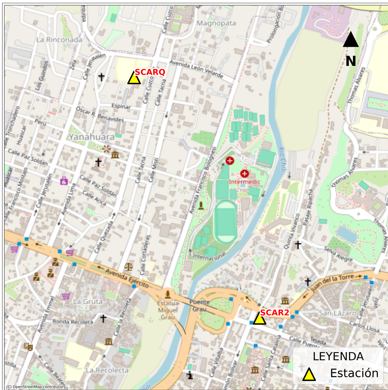
Figura 2: Mapa de ubicación de la(s) estación(es) acelerográfica(s) que registraron el Sismo de Aplao, Castilla - Arequipa del 03 de abril de 2025 a las 20:37:05 (hora local)
