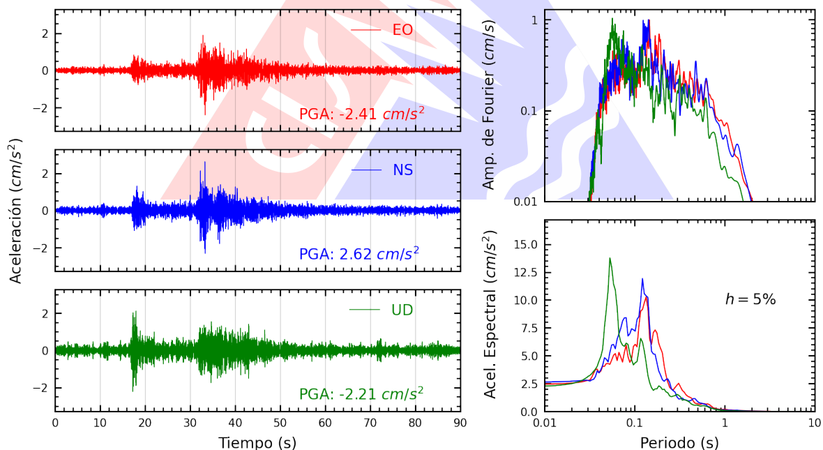
Figura A.2: Registros tiempo-historia, espectros de Fourier y de respuesta en las direcciones EO, NS y UD de la estación SCAR2. Sismo de Aplao, Castilla - Arequipa de 2025-04-03, 20:37:05 (Hora local)
