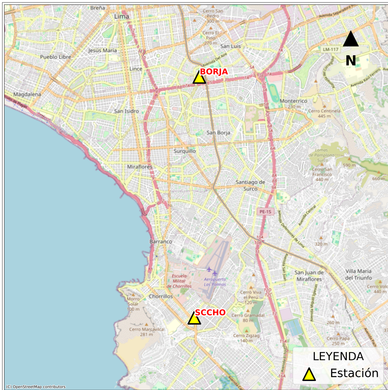
Figura 2: Mapa de ubicación de la(s) estación(es) acelerográfica(s) que registraron el Sismo de Huacho, Huaura - Lima del 03 de abril de 2025 a las 23:45:41 (hora local)
