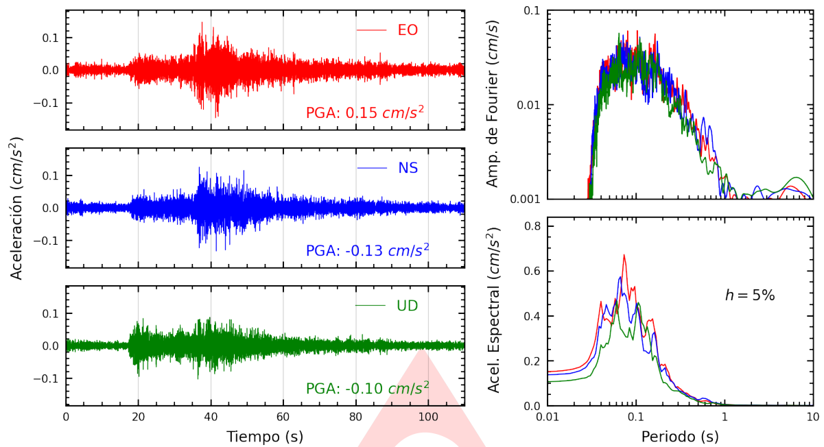
Figura A.1: Registros tiempo-historia, espectros de Fourier y de respuesta en las direcciones EO, NS y UD de la estación BORJA. Sismo de Huacho, Huaura - Lima de 2025-04-03, 23:45:41 (Hora local)
