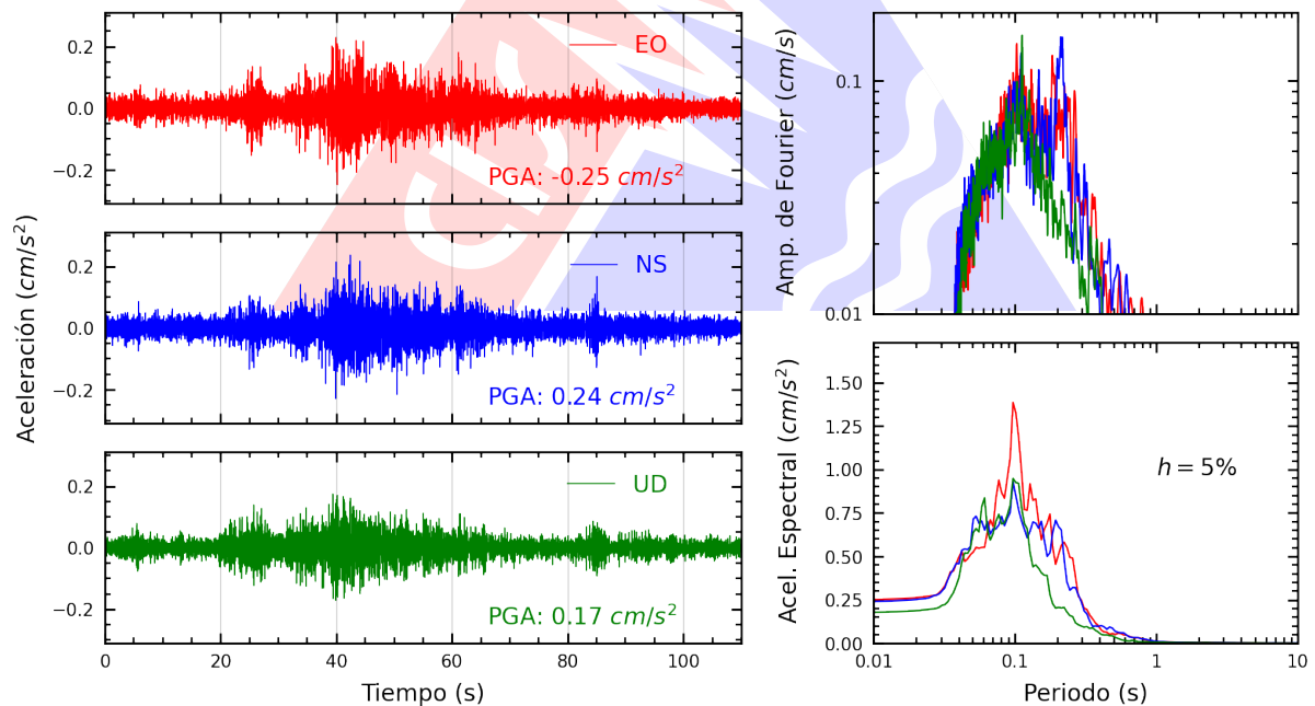
Figura A.2: Registros tiempo-historia, espectros de Fourier y de respuesta en las direcciones EO, NS y UD de la estación SCCHO. Sismo de Huacho, Huaura - Lima de 2025-04-03, 23:45:41 (Hora local)
