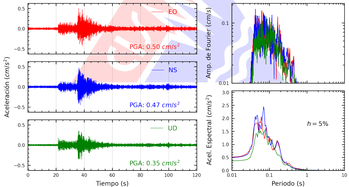
Figura A.2: Registros tiempo-historia, espectros de Fourier y de respuesta en las direcciones EO, NS y UD de la estación BORJA. Sismo de Calango, Cañete - Lima de 2025-04-07, 10:24:02 (Hora local)
