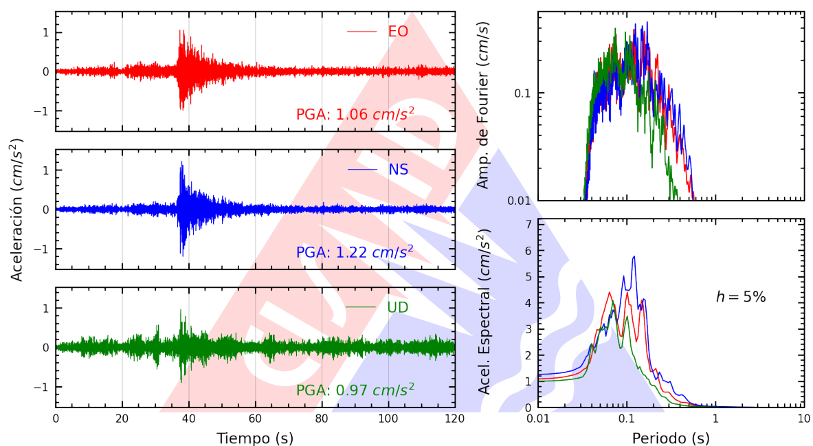
Figura A.3: Registros tiempo-historia, espectros de Fourier y de respuesta en las direcciones EO, NS y UD de la estación SCOLI. Sismo de Calango, Cañete - Lima de 2025-04-07, 10:24:02 (Hora local)
