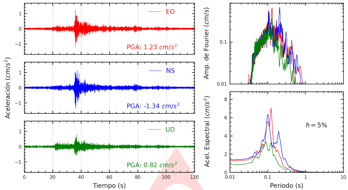
Figura A.1: Registros tiempo-historia, espectros de Fourier y de respuesta en las direcciones EO, NS y UD de la estación SCCHO. Sismo de Calango, Cañete - Lima de 2025-04-07, 10:24:02 (Hora local)
