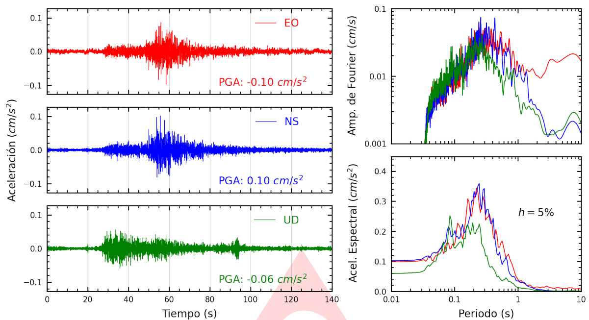
Figura A.1: Registros tiempo-historia, espectros de Fourier y de respuesta en las direcciones EO, NS y UD de la estación SCCHI. Sismo de Paita, Paita - Piura de 2025-04-07, 07:17:14 (Hora local)
