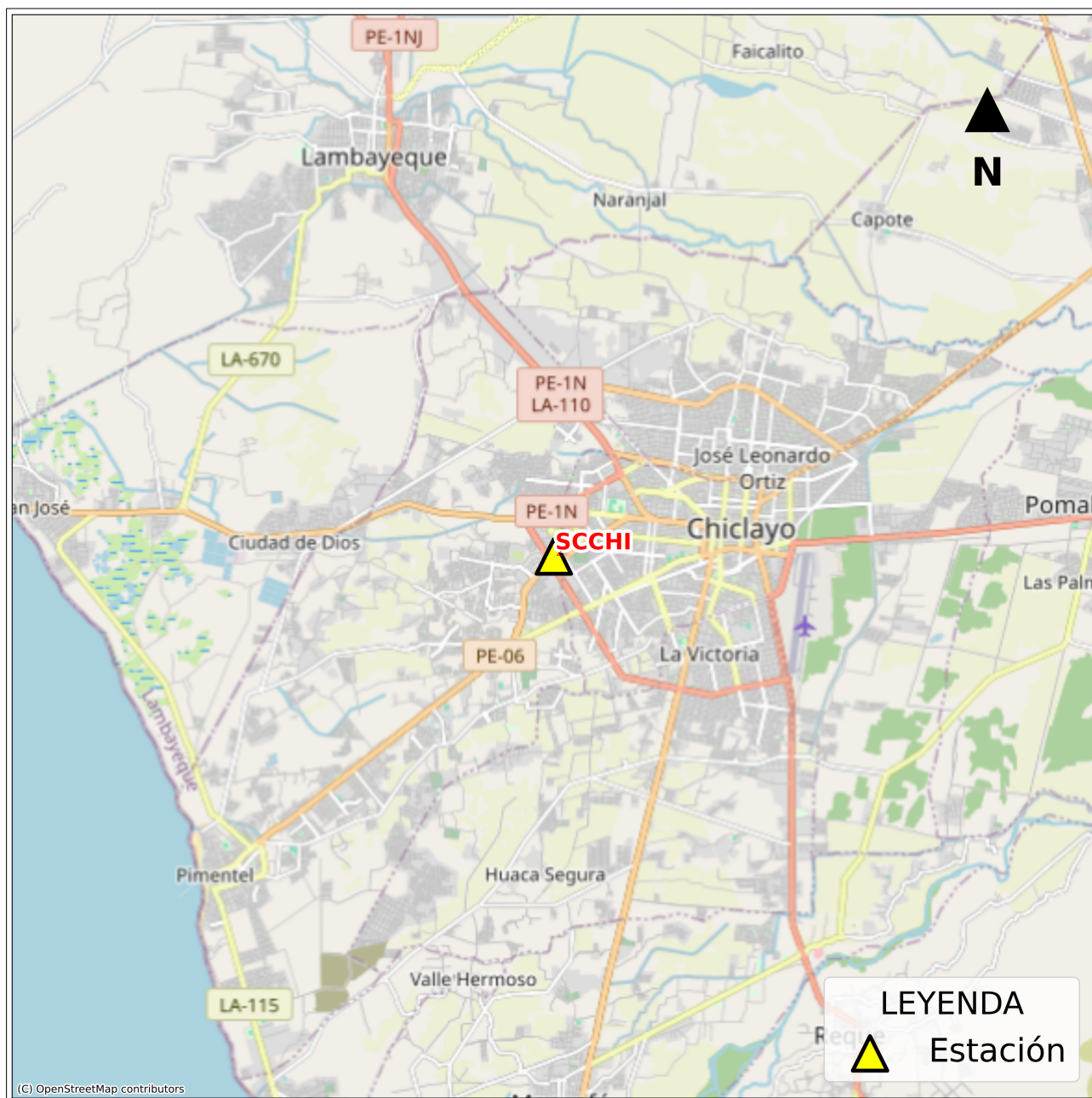
Figura 2: Mapa de ubicación de la(s) estación(es) acelerográfica(s) que registraron el Sismo de Paita, Paita - Piura del 07 de abril de 2025 a las 07:17:14 (hora local)
