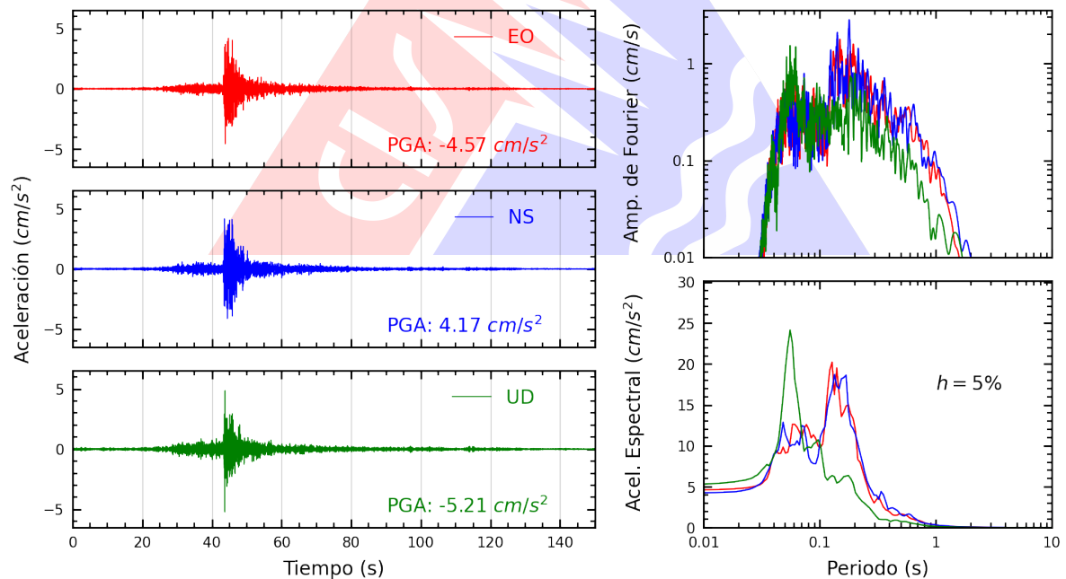
Figura A.2: Registros tiempo-historia, espectros de Fourier y de respuesta en las direcciones EO, NS y UD de la estación SCAR2. Sismo de Camana, Camana - Arequipa de 2025-04-08, 03:43:27 (Hora local)
