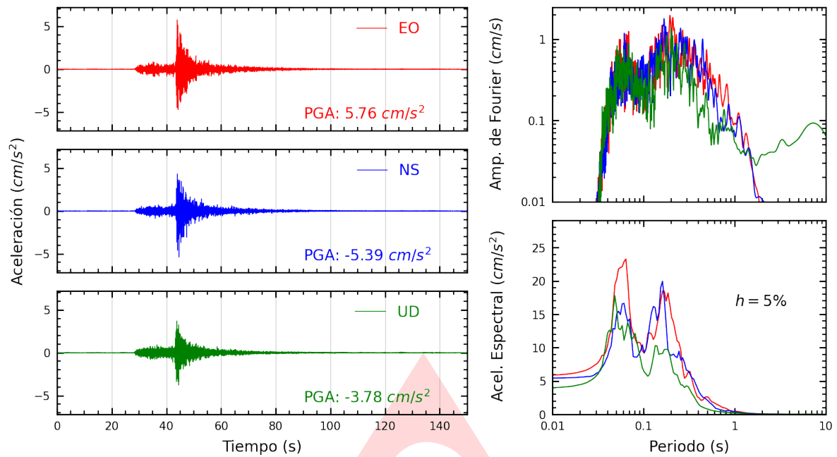
Figura A.1: Registros tiempo-historia, espectros de Fourier y de respuesta en las direcciones EO, NS y UD de la estación SCARQ. Sismo de Camana, Camana - Arequipa de 2025-04-08, 03:43:27 (Hora local)
