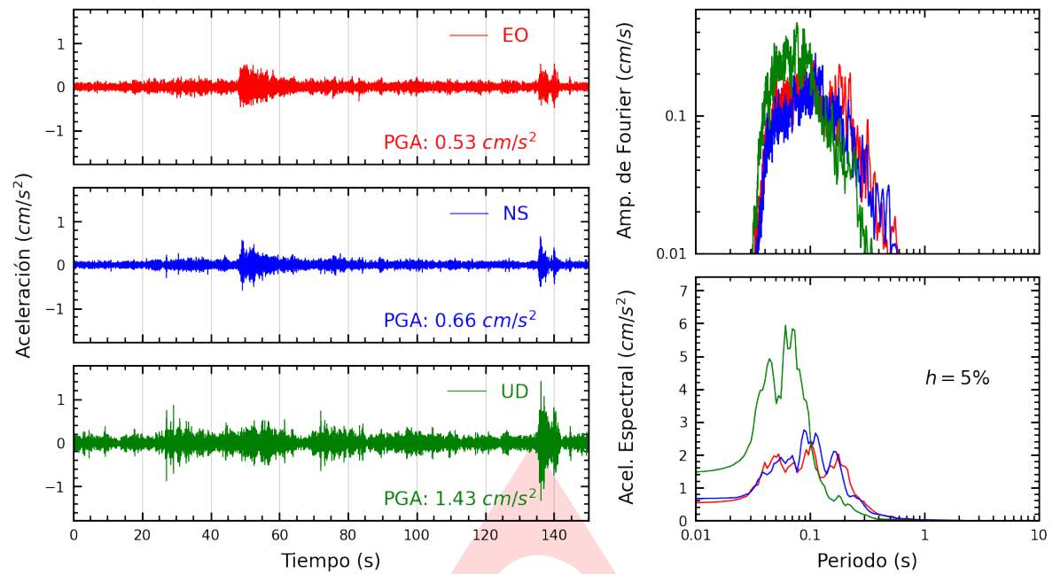
Figura A.1: Registros tiempo-historia, espectros de Fourier y de respuesta en las direcciones EO, NS y UD de la estación SCOLI. Sismo de Oyon, Oyon - Lima de 2025-04-09, 11:37:54 (Hora local)
