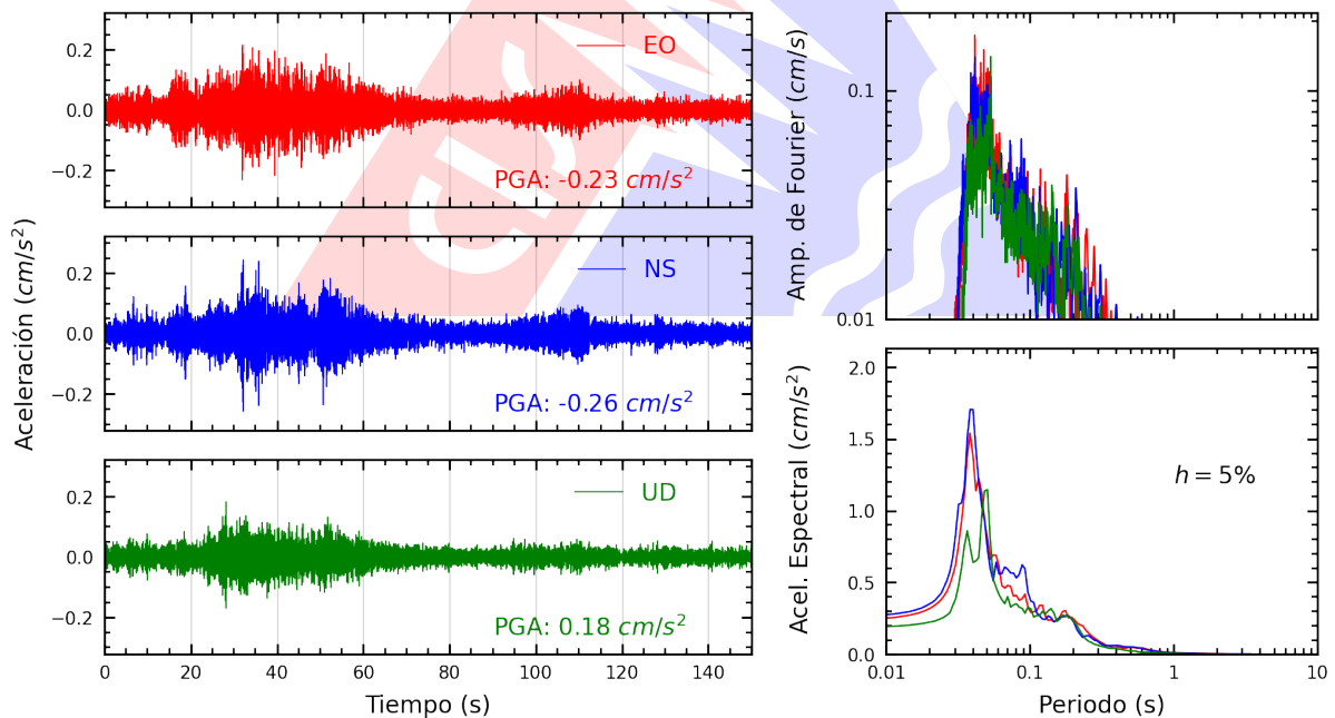
Figura A.2: Registros tiempo-historia, espectros de Fourier y de respuesta en las direcciones EO, NS y UD de la estación BORJA. Sismo de Oyon, Oyon - Lima de 2025-04-09, 11:37:54 (Hora local)
