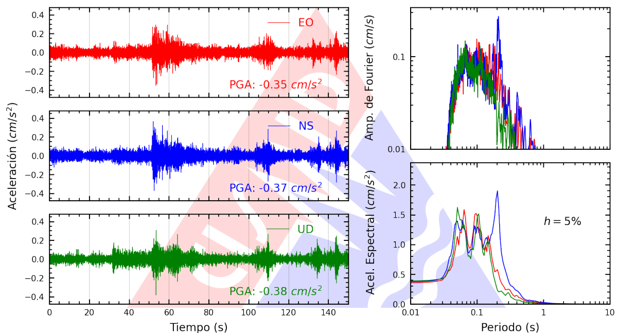
Figura A.3: Registros tiempo-historia, espectros de Fourier y de respuesta en las direcciones EO, NS y UD de la estación SCCHO. Sismo de Oyon, Oyon - Lima de 2025-04-09, 11:37:54 (Hora local)
