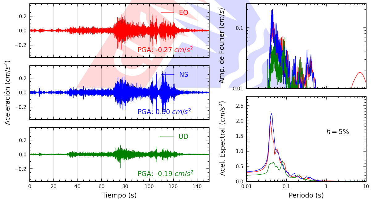
Figura A.2: Registros tiempo-historia, espectros de Fourier y de respuesta en las direcciones EO, NS y UD de la estación SCTRU. Sismo de Sechura, Sechura - Piura de 2025-04-09, 02:40:37 (Hora local)
