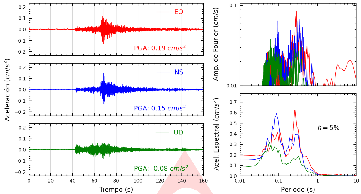
Figura A.1: Registros tiempo-historia, espectros de Fourier y de respuesta en las direcciones EO, NS y UD de la estación SCCHI. Sismo de Sechura, Sechura - Piura de 2025-04-09, 02:40:37 (Hora local)
