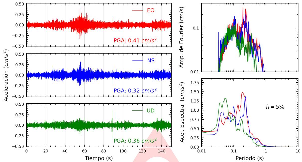
Figura A.1: Registros tiempo-historia, espectros de Fourier y de respuesta en las direcciones EO, NS y UD de la estación SCCHO. Sismo de Chuschi, Cangallo - Ayacucho de 2025-04-10, 12:13:14 (Hora local)
