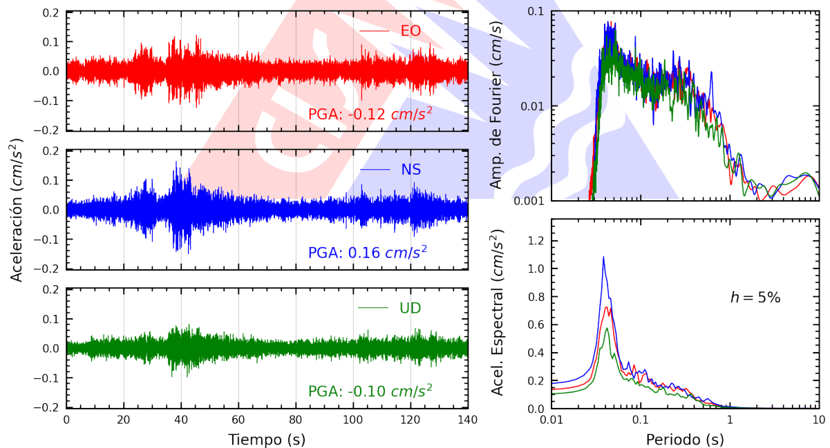
Figura A.2: Registros tiempo-historia, espectros de Fourier y de respuesta en las direcciones EO, NS y UD de la estación BORJA. Sismo de Chuschi, Cangallo - Ayacucho de 2025-04-10, 12:13:14 (Hora local)
