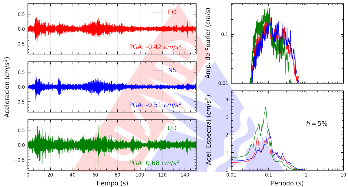
Figura A.3: Registros tiempo-historia, espectros de Fourier y de respuesta en las direcciones EO, NS y UD de la estación SCOLI. Sismo de Chuschi, Cangallo - Ayacucho de 2025-04-10, 12:13:14 (Hora local)
