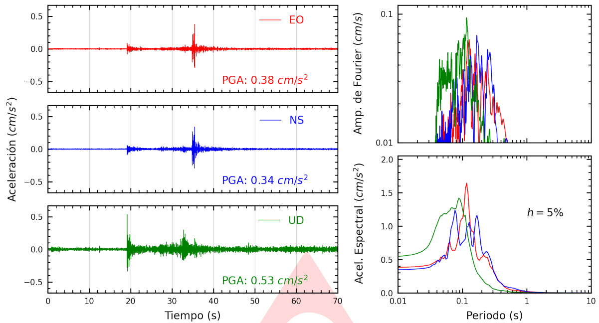
Figura A.1: Registros tiempo-historia, espectros de Fourier y de respuesta en las direcciones EO, NS y UD de la estación SCPUC. Sismo de Curimana, Padre Abad - Ucayali de 2025-04-12, 20:58:59 (Hora local)
