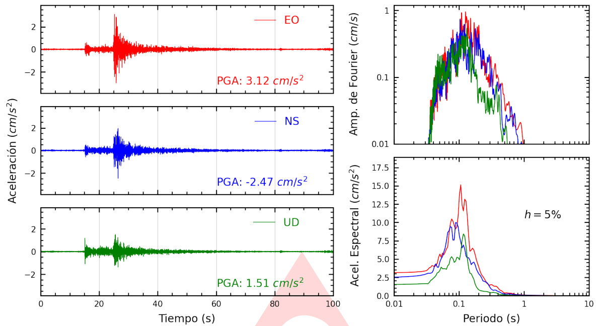
Figura A.1: Registros tiempo-historia, espectros de Fourier y de respuesta en las direcciones EO, NS y UD de la estación SCCHO. Sismo de Mala, Cañete - Lima de 2025-04-12, 22:47:00 (Hora local)
