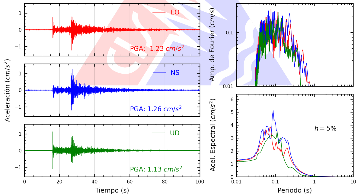
Figura A.2: Registros tiempo-historia, espectros de Fourier y de respuesta en las direcciones EO, NS y UD de la estación BORJA. Sismo de Mala, Cañete - Lima de 2025-04-12, 22:47:00 (Hora local)
