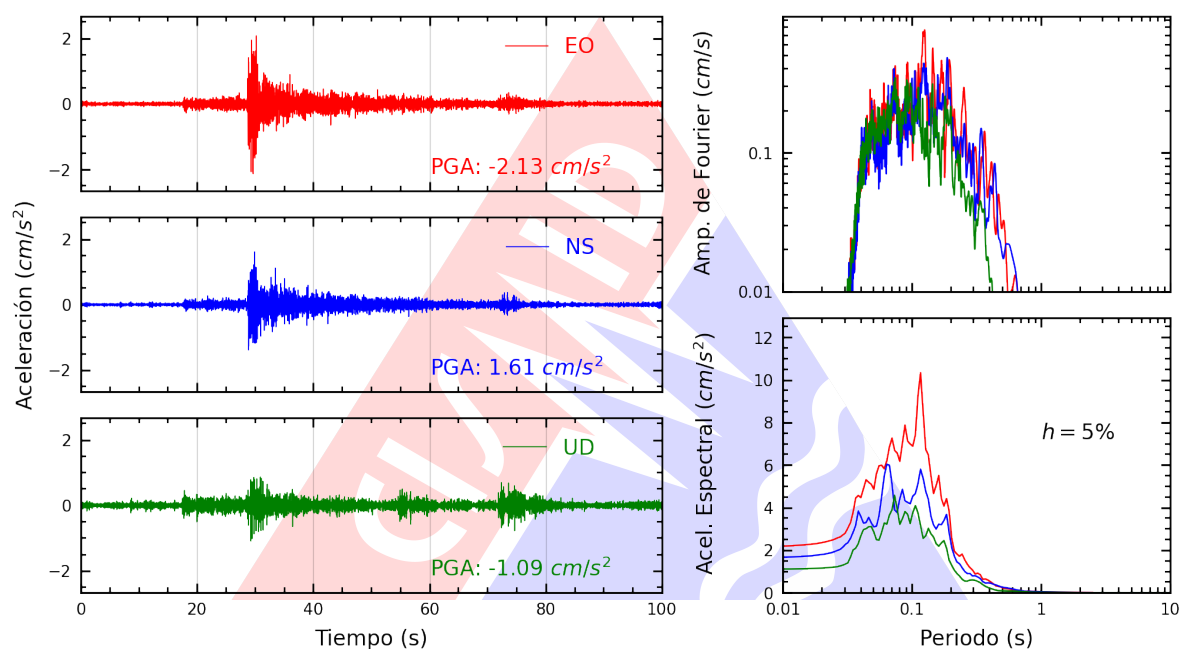
Figura A.3: Registros tiempo-historia, espectros de Fourier y de respuesta en las direcciones EO, NS y UD de la estación SCOLI. Sismo de Mala, Cañete - Lima de 2025-04-12, 22:47:00 (Hora local)
