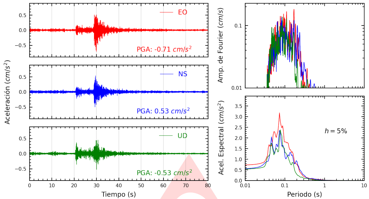
Figura A.1: Registros tiempo-historia, espectros de Fourier y de respuesta en las direcciones EO, NS y UD de la estación SCCHO. Sismo de Chilca, Cañete - Lima de 2025-04-13, 03:03:29 (Hora local)
