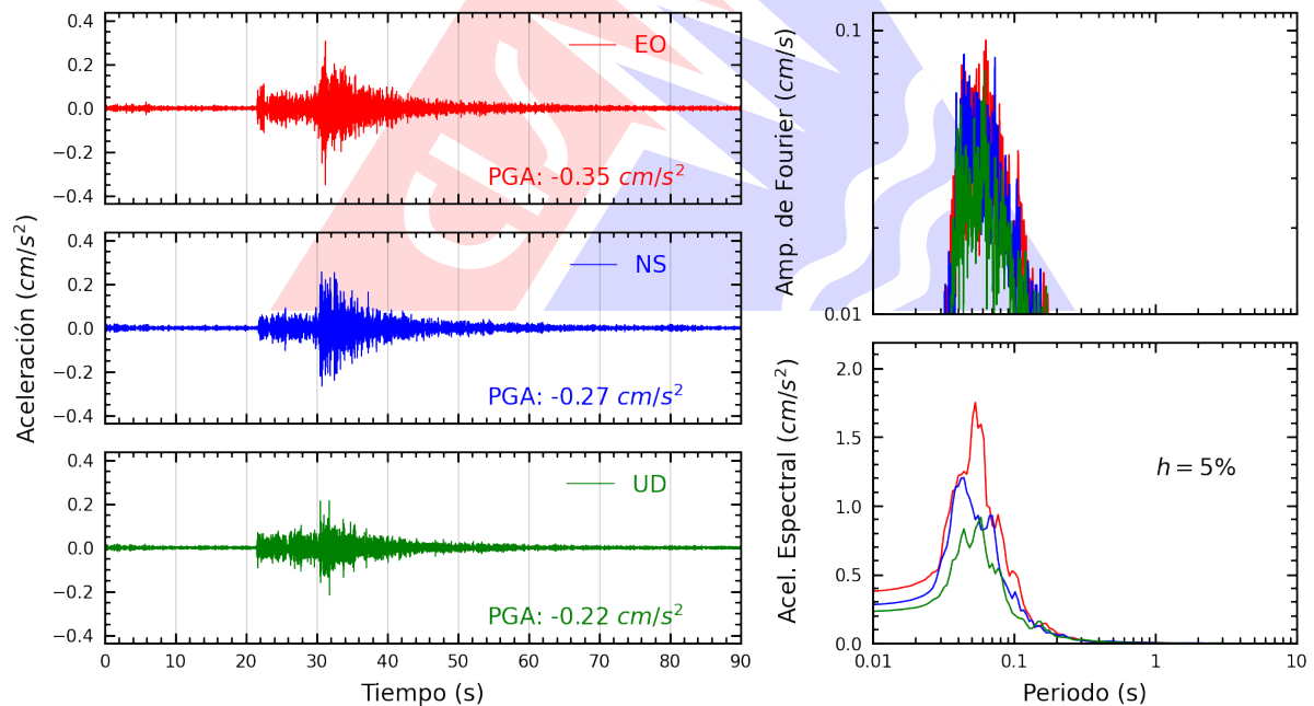
Figura A.2: Registros tiempo-historia, espectros de Fourier y de respuesta en las direcciones EO, NS y UD de la estación BORJA. Sismo de Chilca, Cañete - Lima de 2025-04-13, 03:03:29 (Hora local)
