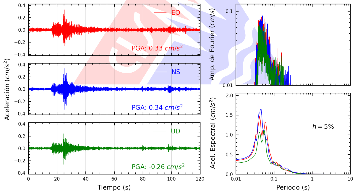
Figura A.2: Registros tiempo-historia, espectros de Fourier y de respuesta en las direcciones EO, NS y UD de la estación BORJA. Sismo de Chilca, Cañete - Lima de 2025-04-17, 05:10:55 (Hora local)
