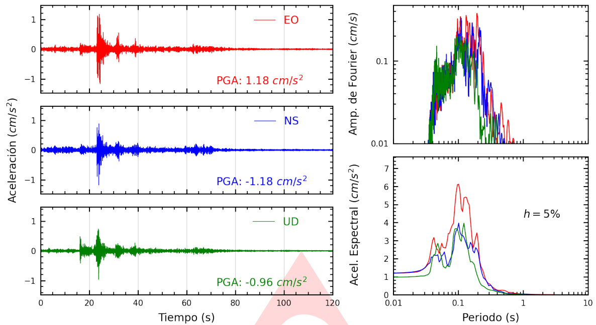
Figura A.1: Registros tiempo-historia, espectros de Fourier y de respuesta en las direcciones EO, NS y UD de la estación SCCHO. Sismo de Chilca, Cañete - Lima de 2025-04-17, 05:10:55 (Hora local)
