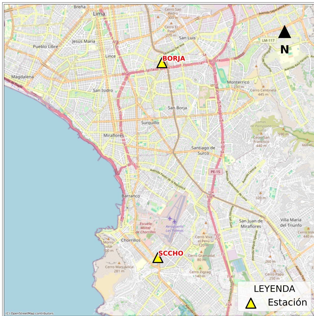
Figura 2: Mapa de ubicación de la(s) estación(es) acelerográfica(s) que registraron el Sismo de Chilca, Cañete - Lima del 17 de abril de 2025 a las 05:10:55 (hora local)
