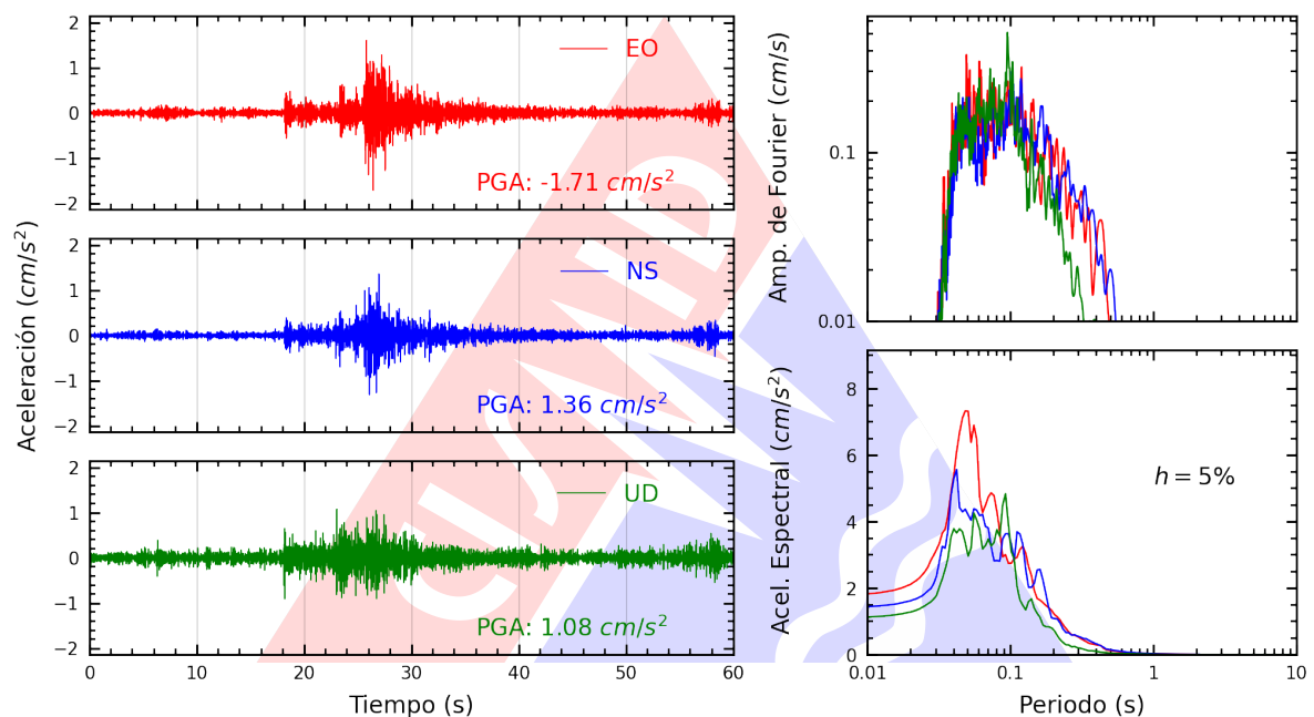
Figura A.3: Registros tiempo-historia, espectros de Fourier y de respuesta en las direcciones EO, NS y UD de la estación SCOLI. Sismo de Chilca, Cañete - Lima de 2025-04-25, 16:21:07 (Hora local)
