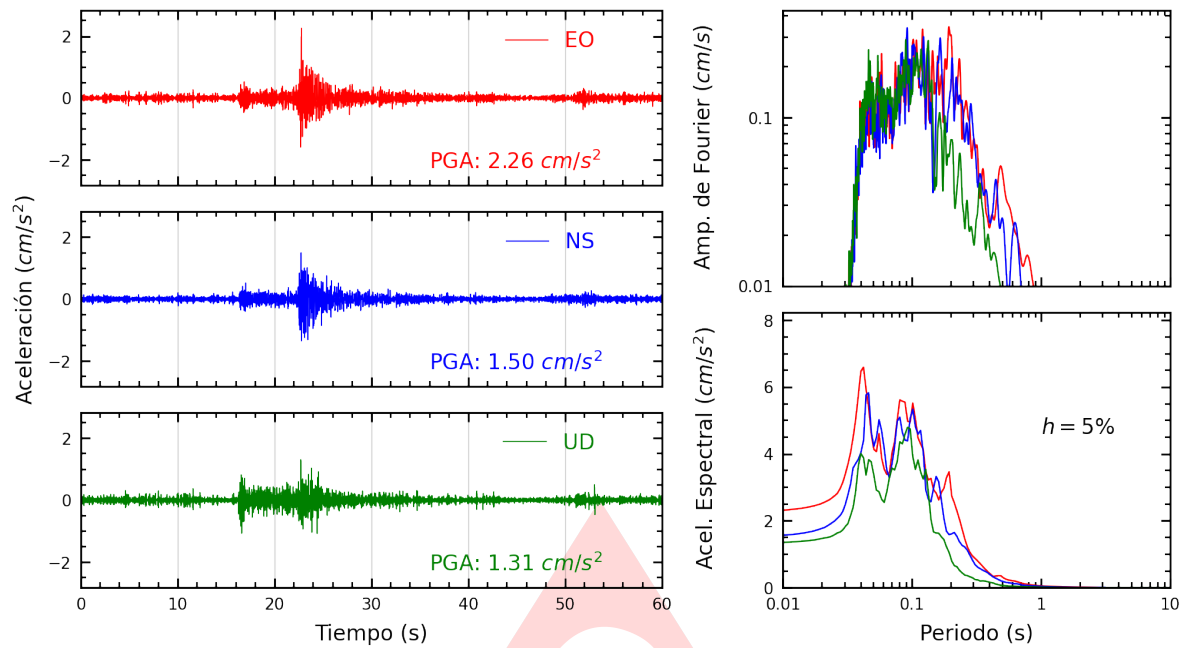
Figura A.1: Registros tiempo-historia, espectros de Fourier y de respuesta en las direcciones EO, NS y UD de la estación SCCHO. Sismo de Chilca, Cañete - Lima de 2025-04-25, 16:21:07 (Hora local)
