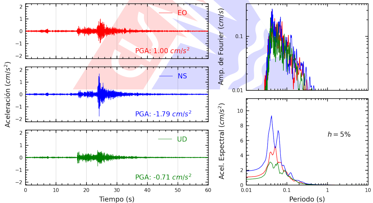
Figura A.2: Registros tiempo-historia, espectros de Fourier y de respuesta en las direcciones EO, NS y UD de la estación BORJA. Sismo de Chilca, Cañete - Lima de 2025-04-25, 16:21:07 (Hora local)
