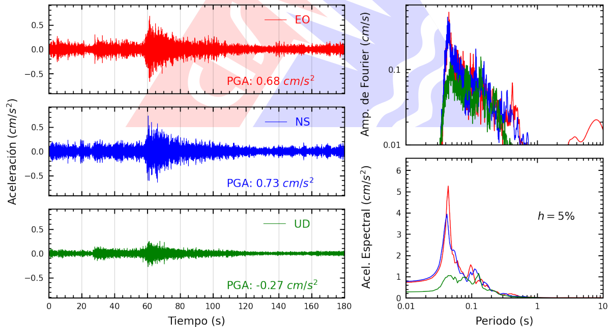
Figura A.2: Registros tiempo-historia, espectros de Fourier y de respuesta en las direcciones EO, NS y UD de la estación SCTRU. Sismo de Huancabamba, Huancabamba - Piura de 2025-04-25, 21:40:22 (Hora local)
