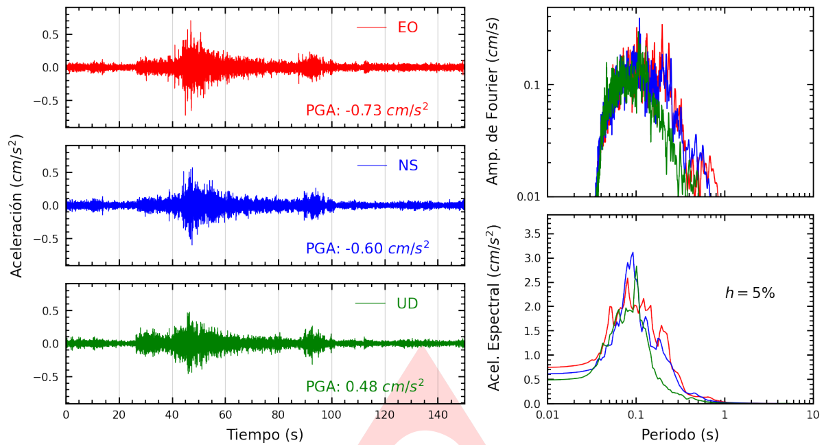
Figura A.1: Registros tiempo-historia, espectros de Fourier y de respuesta en las direcciones EO, NS y UD de la estación SCCHO. Sismo de Chinchá Alta, Chinchá - Ica de 2025-04-26, 13:56:02 (Hora local)
