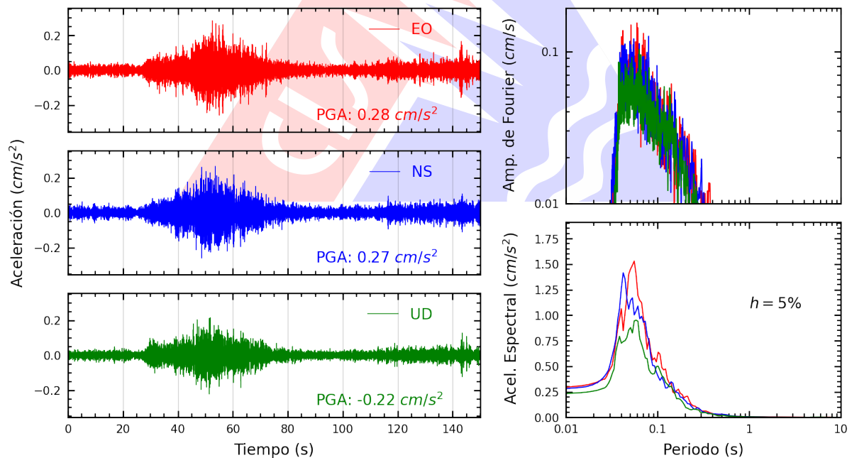
Figura A.2: Registros tiempo-historia, espectros de Fourier y de respuesta en las direcciones EO, NS y UD de la estación BORJA. Sismo de Chinchá Alta, Chinchá - Ica de 2025-04-26, 13:56:02 (Hora local)
