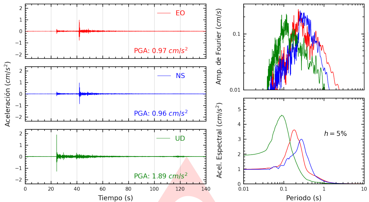
Figura A.1: Registros tiempo-historia, espectros de Fourier y de respuesta en las direcciones EO, NS y UD de la estación SCPUC. Sismo de Pucallpa, Coronel Portillo - Ucayali de 2025-04-27, 04:38:38 (Hora local)
