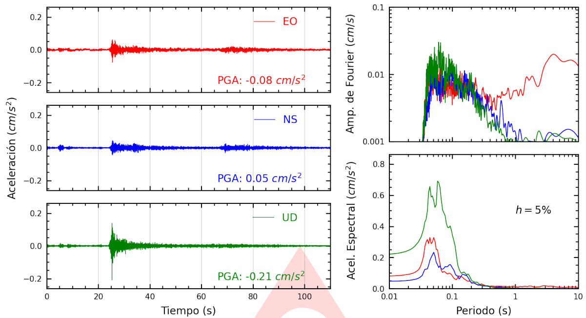
Figura A.1: Registros tiempo-historia, espectros de Fourier y de respuesta en las direcciones EO, NS y UD de la estación SCCHI. Sismo de Sta. Maria De Nieva, Condorcanqui - Amazonas de 2025-04-30, 01:46:18 (Hora local)
