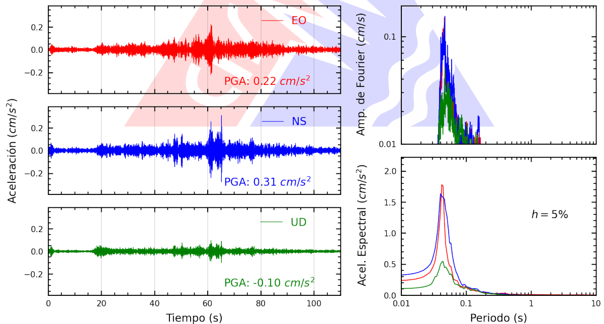
Figura A.2: Registros tiempo-historia, espectros de Fourier y de respuesta en las direcciones EO, NS y UD de la estación SCTRU. Sismo de Sta. Maria De Nieva, Condorcanqui - Amazonas de 2025-04-30, 01:46:18 (Hora local)
