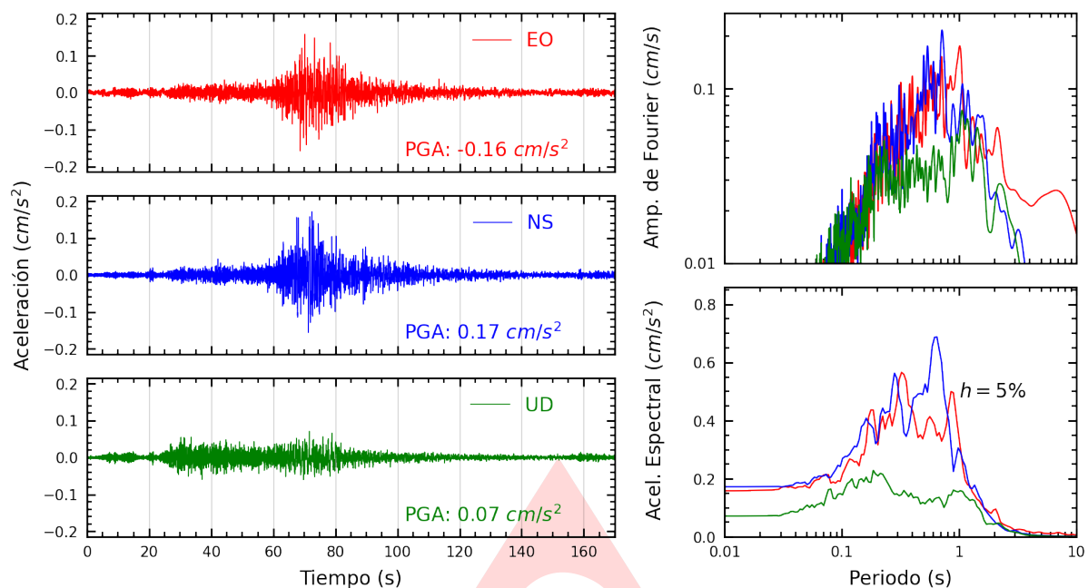
Figura A.1: Registros tiempo-historia, espectros de Fourier y de respuesta en las direcciones EO, NS y UD de la estación SCCHI. Sismo de Mancora, Talara - Piura de 2025-05-10, 20:29:52 (Hora local)
