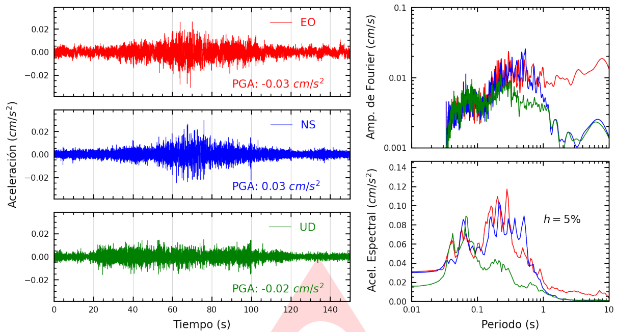
Figura A.1: Registros tiempo-historia, espectros de Fourier y de respuesta en las direcciones EO, NS y UD de la estación SCCHI. Sismo de Mancora, Talara - Piura de 2025-05-10, 21:59:30 (Hora local)
