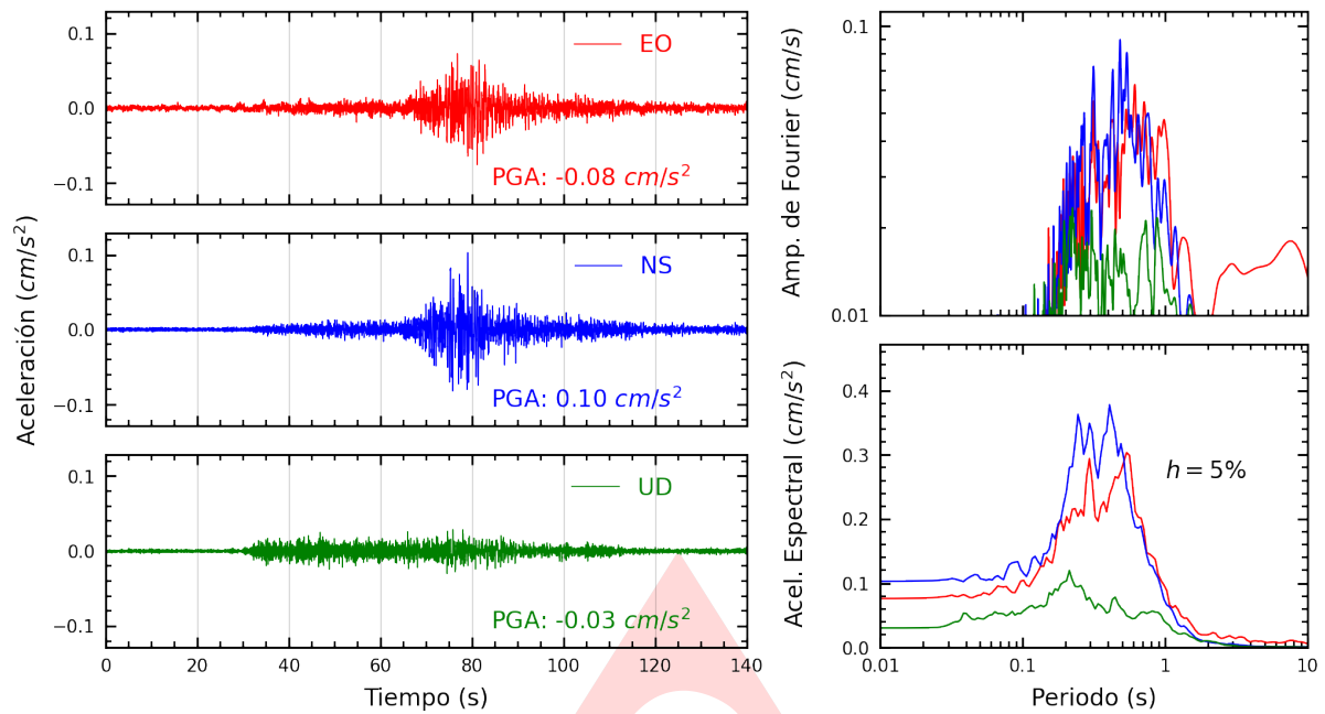
Figura A.1: Registros tiempo-historia, espectros de Fourier y de respuesta en las direcciones EO, NS y UD de la estación SCCHI. Sismo de Mancora, Talara - Piura de 2025-05-11, 00:42:42 (Hora local)
