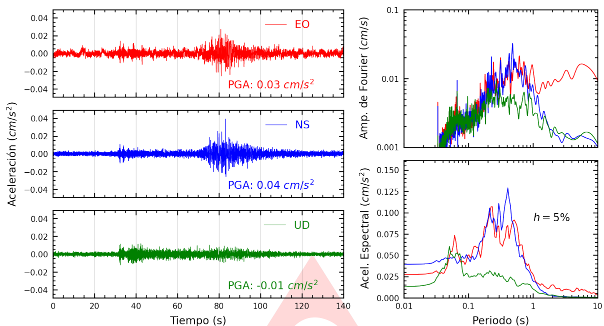
Figura A.1: Registros tiempo-historia, espectros de Fourier y de respuesta en las direcciones EO, NS y UD de la estación SCCHI. Sismo de Mancora, Talara - Piura de 2025-05-11, 00:53:45 (Hora local)
