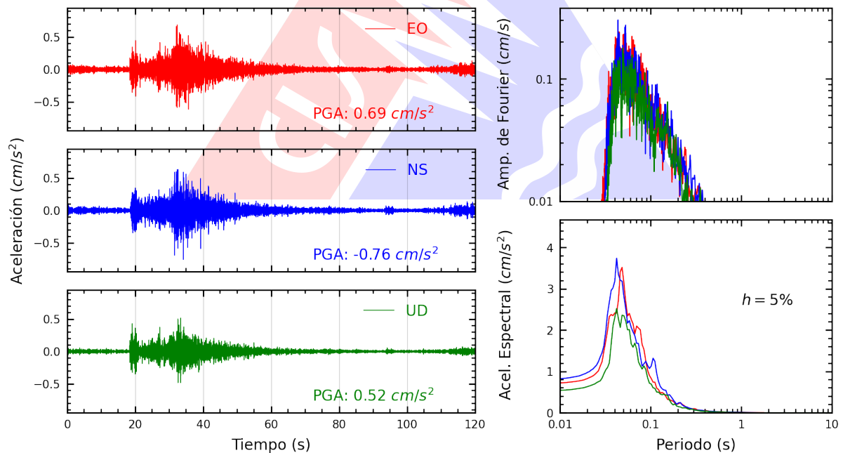
Figura A.2: Registros tiempo-historia, espectros de Fourier y de respuesta en las direcciones EO, NS y UD de la estación BORJA. Sismo de Mala, Cañete - Lima de 2025-05-11, 06:44:40 (Hora local)
