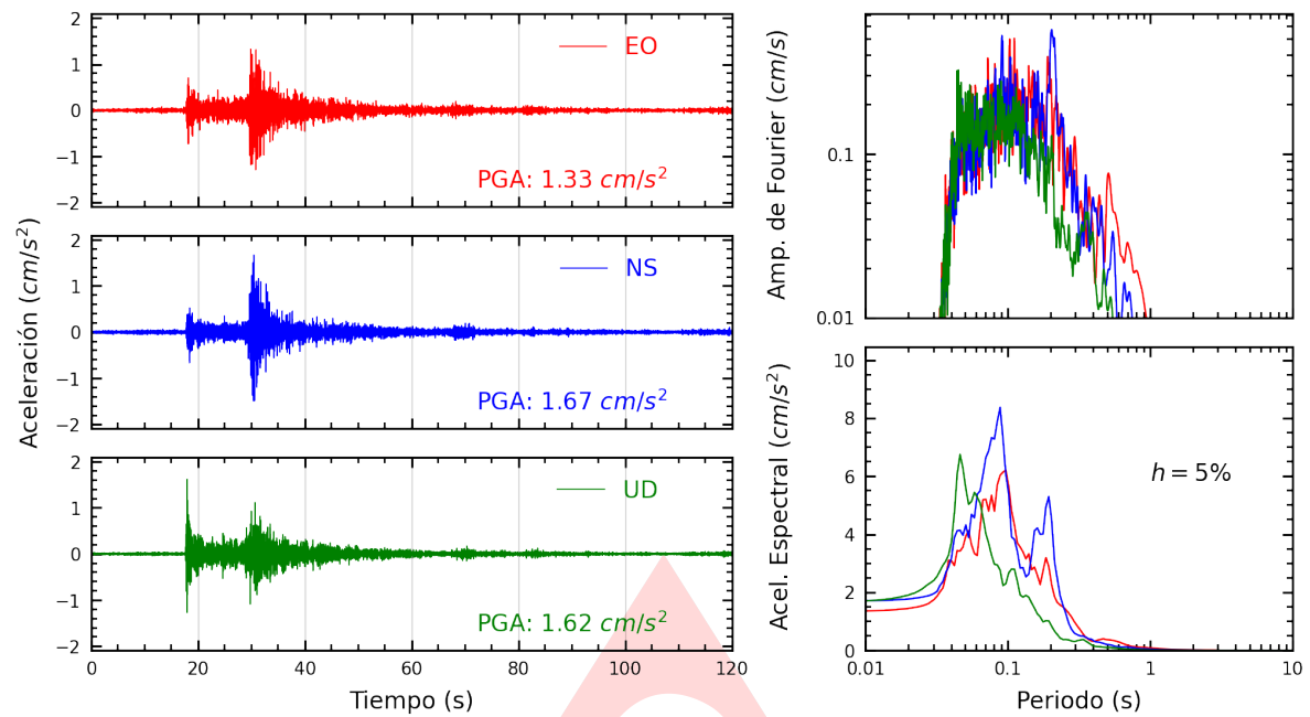
Figura A.1: Registros tiempo-historia, espectros de Fourier y de respuesta en las direcciones EO, NS y UD de la estación SCCHO. Sismo de Mala, Cañete - Lima de 2025-05-11, 06:44:40 (Hora local)
