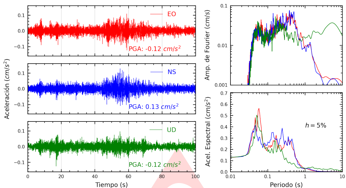
Figura A.1: Registros tiempo-historia, espectros de Fourier y de respuesta en las direcciones EO, NS y UD de la estación SCARQ. Sismo de Chala, Caraveli - Arequipa de 2025-05-11, 01:25:23 (Hora local)
