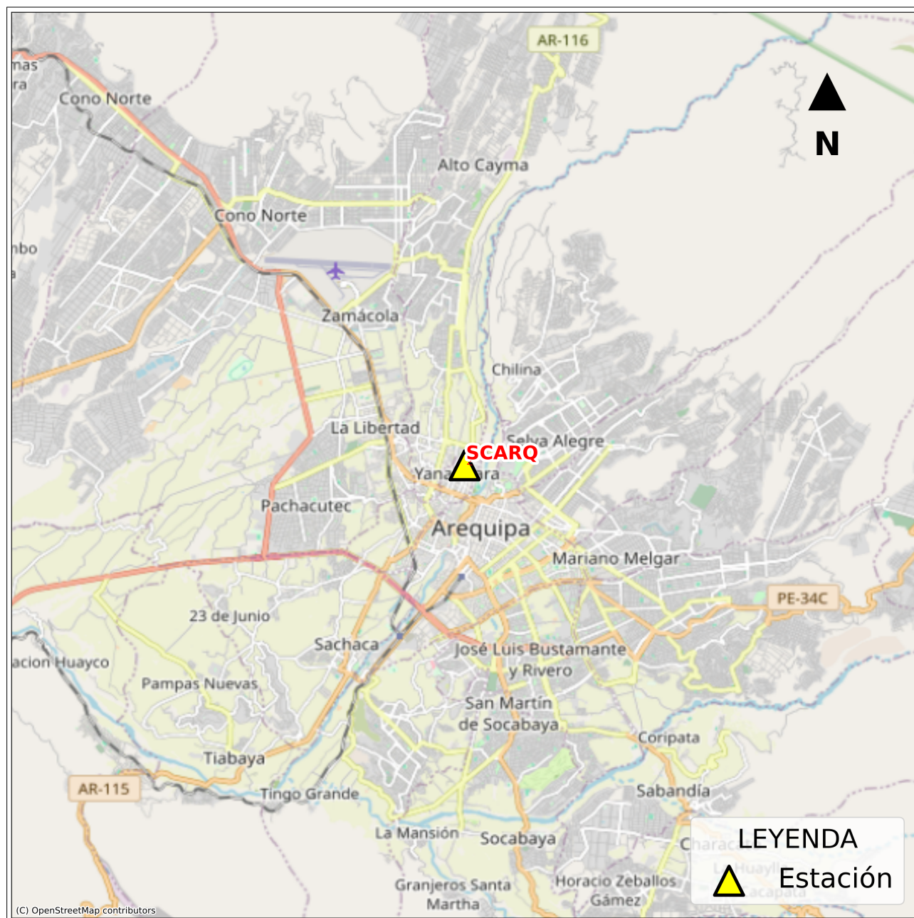
Figura 2: Mapa de ubicación de la(s) estación(es) acelerográfica(s) que registraron el Sismo de Chala, Caraveli - Arequipa del 11 de mayo de 2025 a las 01:25:23 (hora local)
