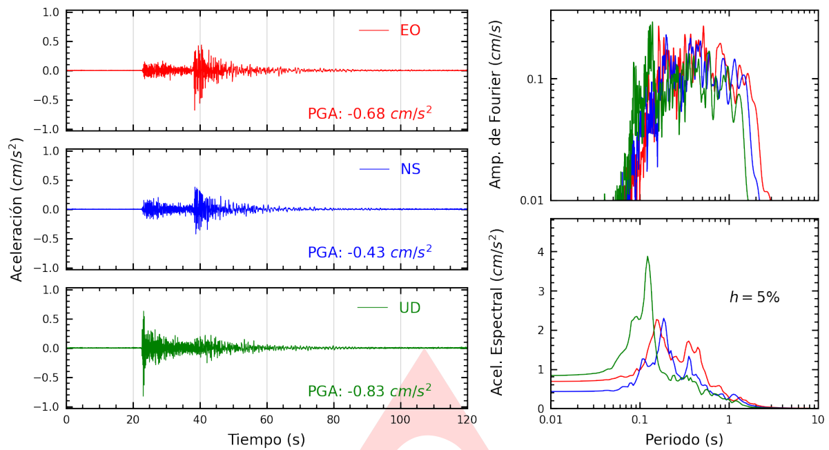
Figura A.1: Registros tiempo-historia, espectros de Fourier y de respuesta en las direcciones EO, NS y UD de la estación SCCUS. Sismo de Santo Tomas, Chumbivilcas - Cusco de 2025-05-13, 02:10:52 (Hora local)
