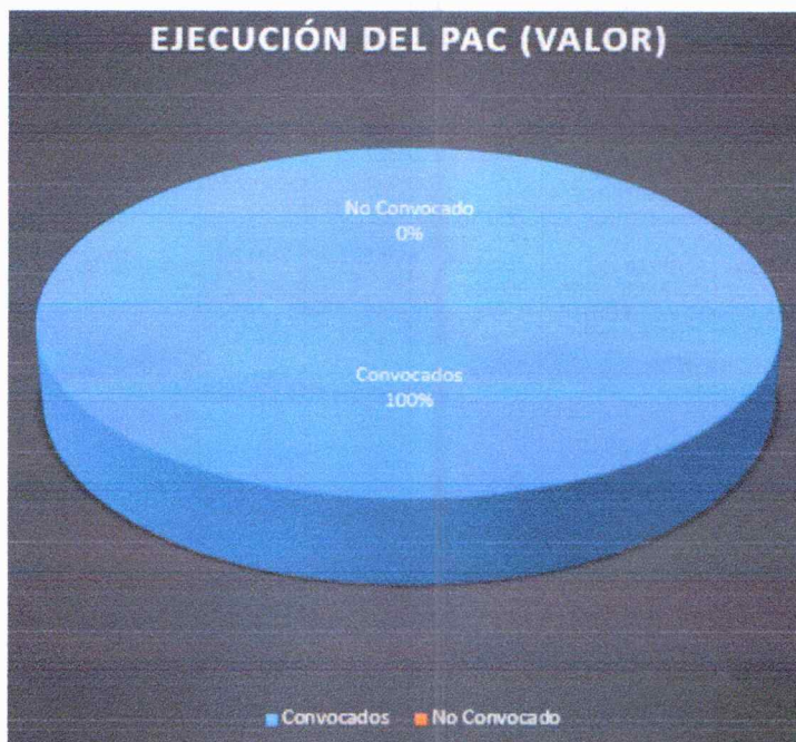
Gráfico N° 6 Resumen de % ejecución PAC 2024 – Cantidades
