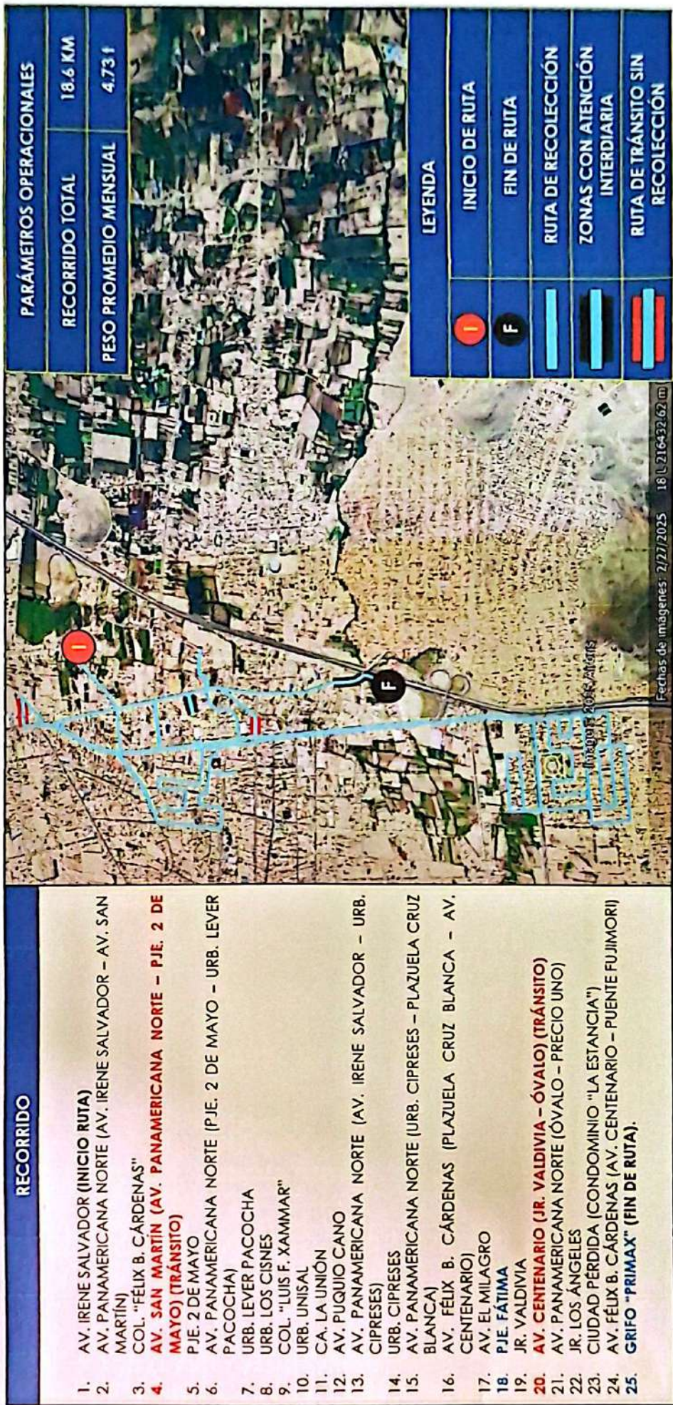
Figura N°. 13. Plano de recorrido operativo - Macro Ruta "Ex Panamericana"
