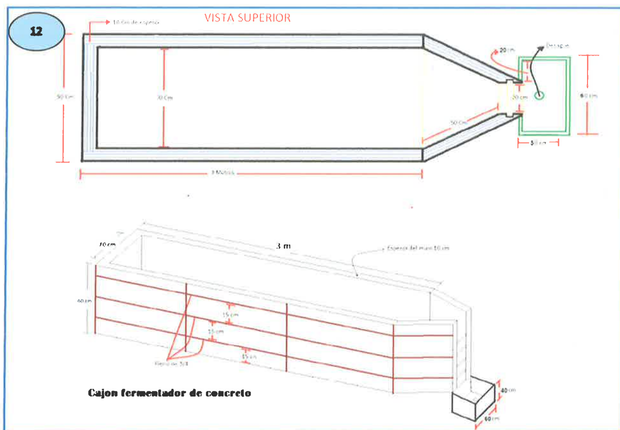
12: Diseño de PBH- Planta de Beneficio Húmedo a implementarse en la comunidad.
