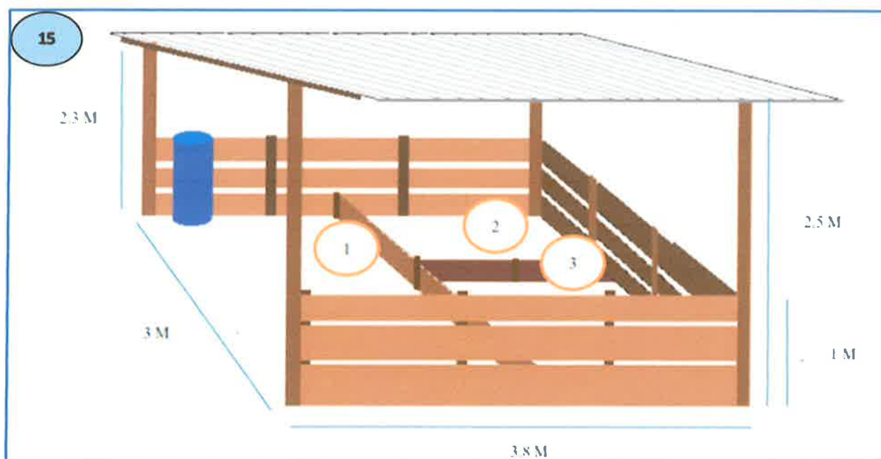
15: Diseño de Compostera a implementarse en la comunidad.
