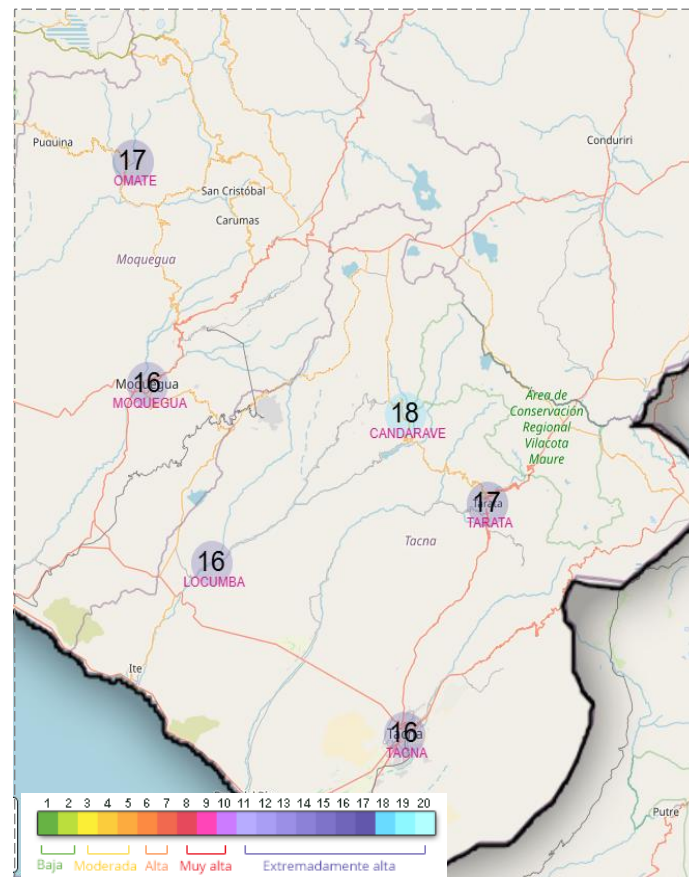
Figura 2: Pronóstico de Índice de radiación UV máximo 20/01/2026
