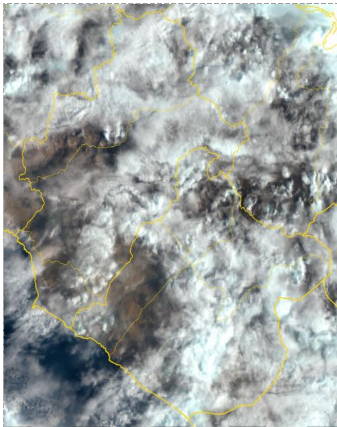
Figura 1: Imagen satelital GOES 19: 19/01/2026 – 08:00 am
