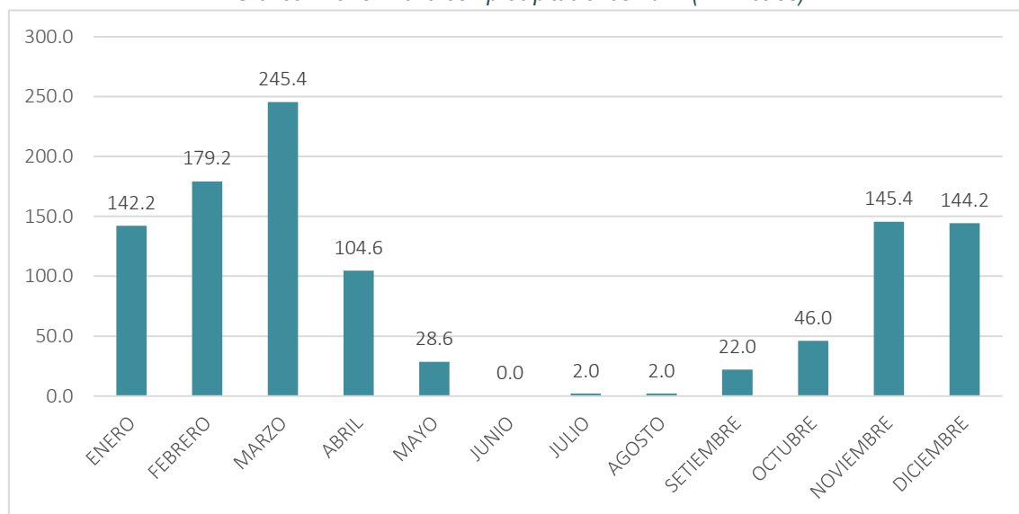
Gráfico 148: Chincheros - precipitaciones 2021 (milímetros)
