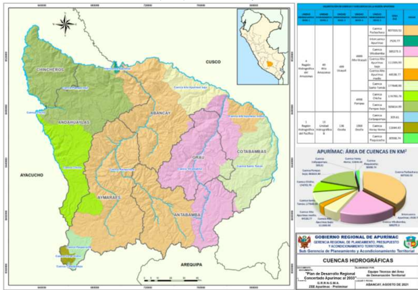
Mapa 25: Apurímac: Cuencas Hidrográficas
