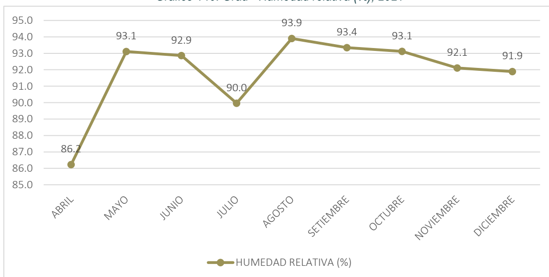
Gráfico 140: Grau - Humedad relativa (%), 2021
