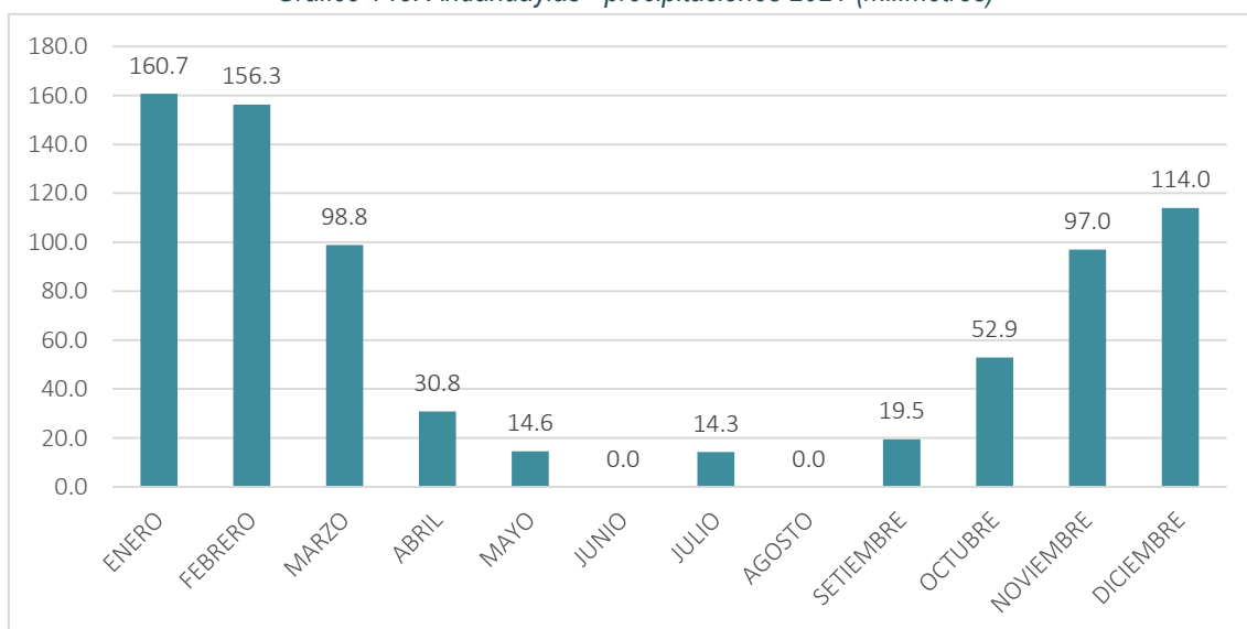
Gráfico 145: Andahuaylas - precipitaciones 2021 (milímetros)
