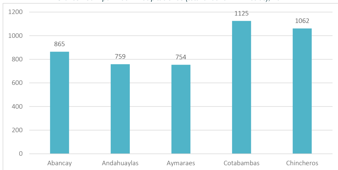
Gráfico 150: Apurímac - Precipitaciones (total anual en milímetros), 2021
