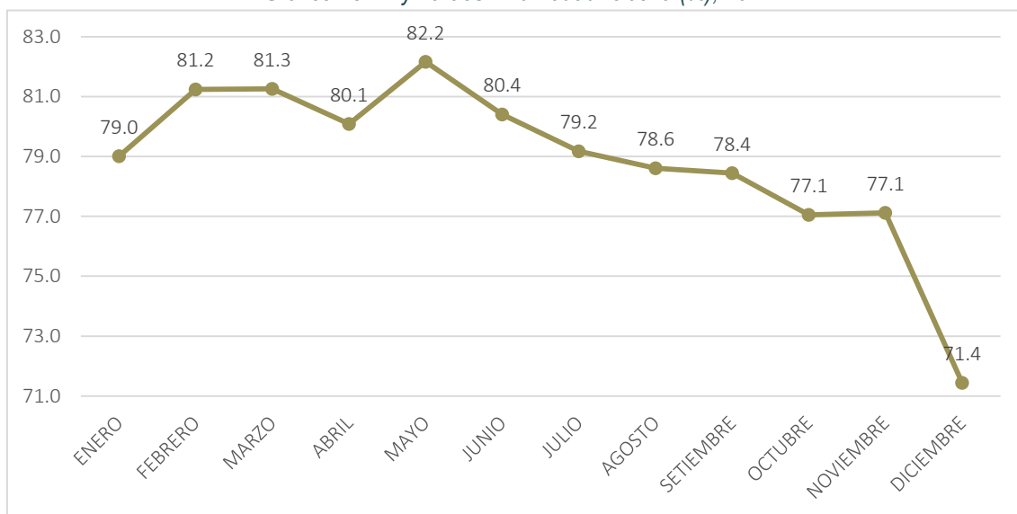
Gráfico 137: Aymaraes - Humedad relativa (%), 2021
