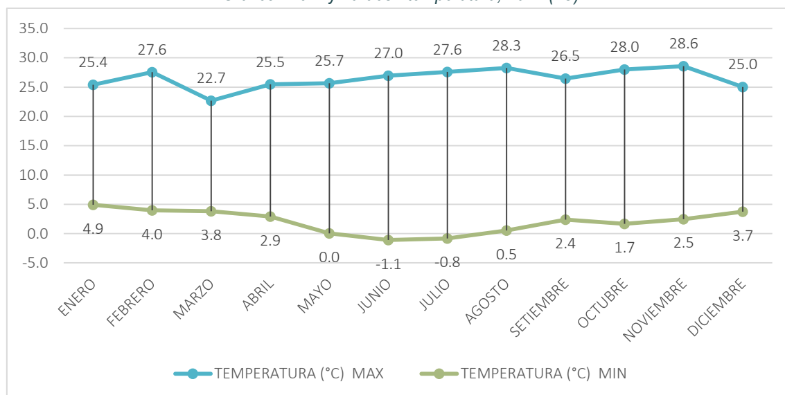
Gráfico 129: Aymaraes - temperatura, 2021 (°C)
