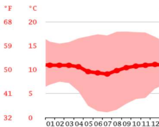
Gráfico 125: Temperatura de Apurímac
