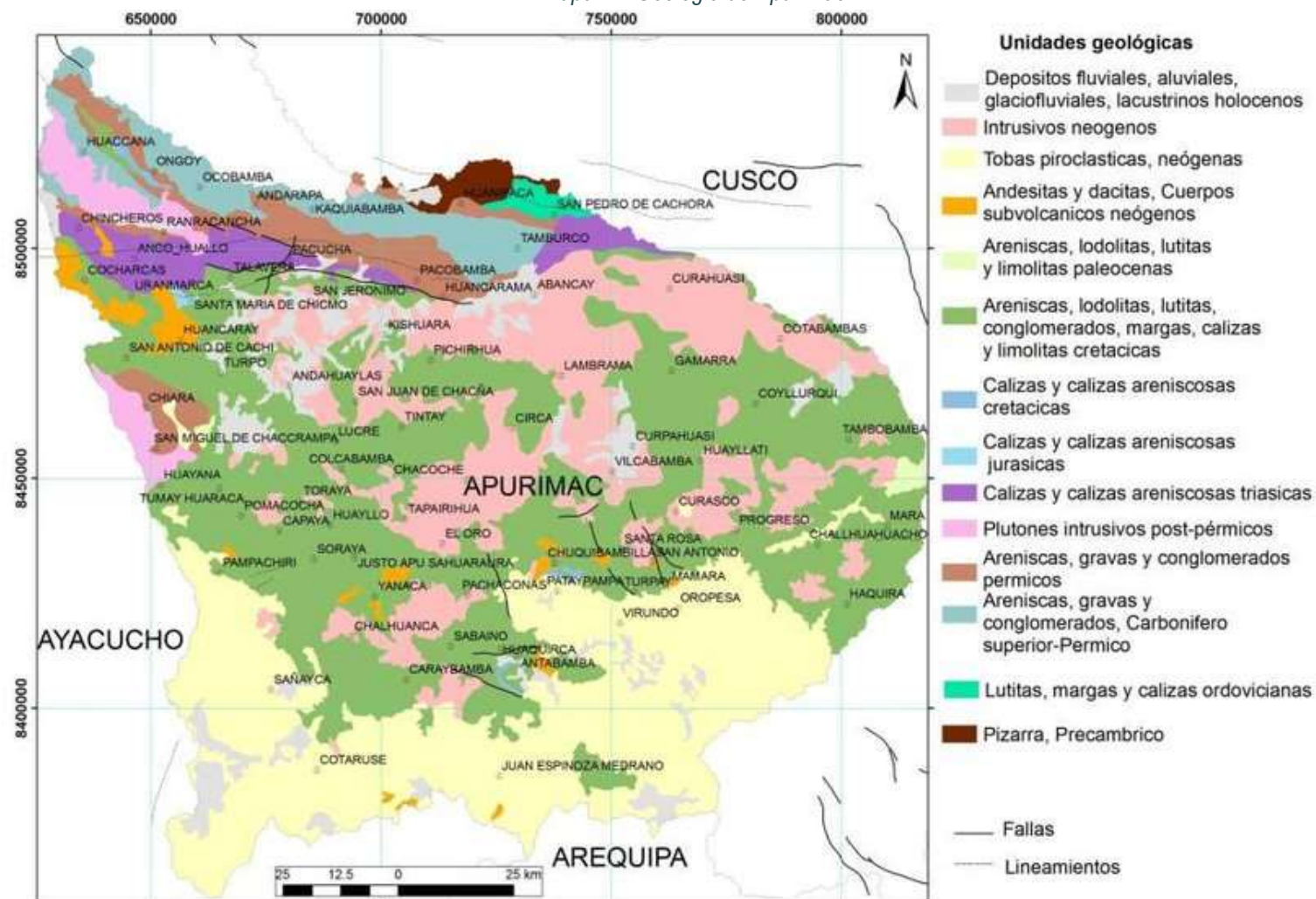
Mapa 24: Geología de Apurímac
