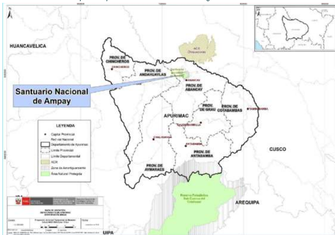
Mapa 34: Apurímac: Áreas Naturales Protegidas en el territorio.
