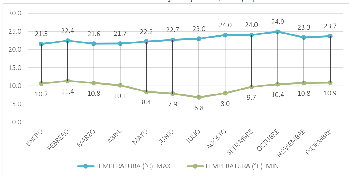
Gráfico 127: Abancay - temperatura, 2021 (°C)
