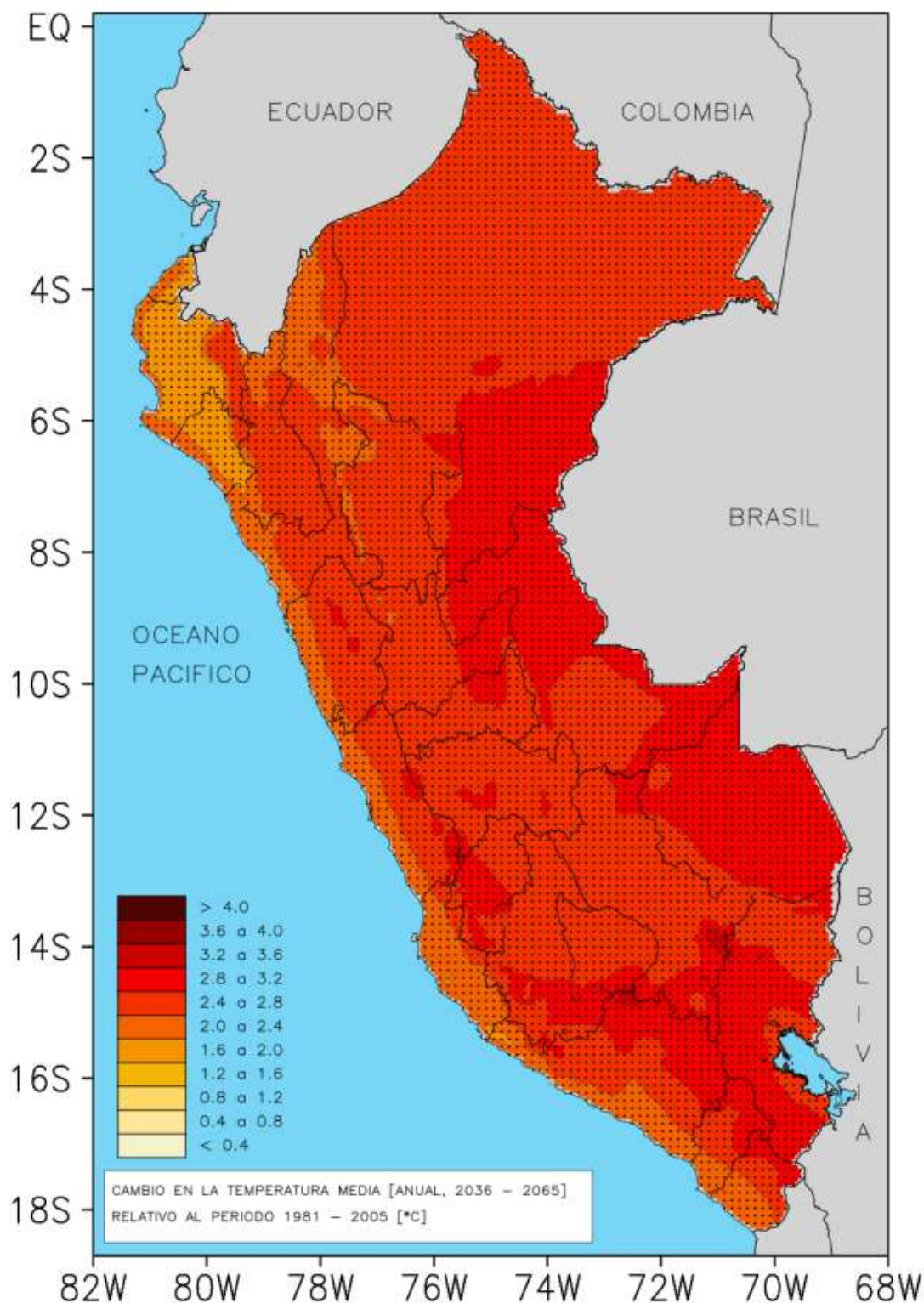
Mapa 57: Cambios en la temperatura media anual centrado al 2050 [°C], respecto al periodo 1981-2005
