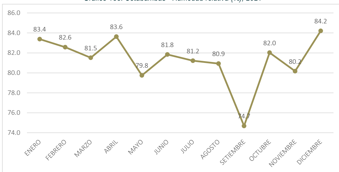
Gráfico 138: Cotabambas - Humedad relativa (%), 2021
