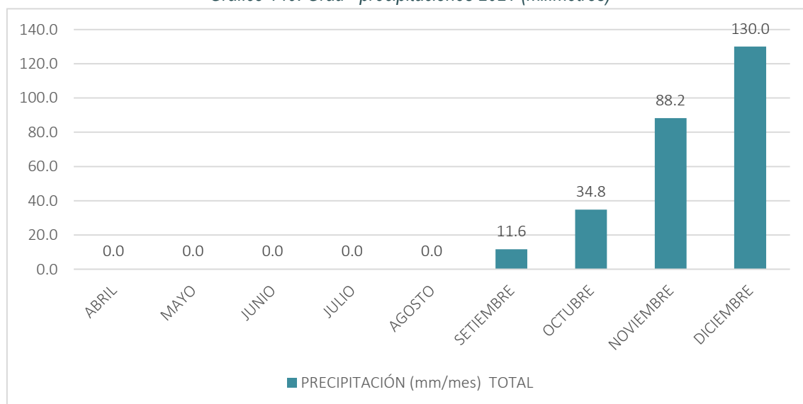
Gráfico 149: Grau - precipitaciones 2021 (milímetros)
