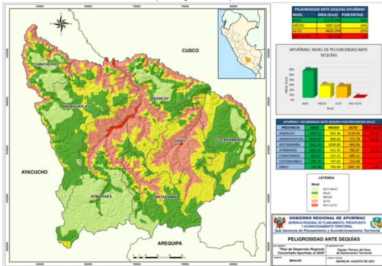
Mapa 46: Peligrosidad ante sequías
