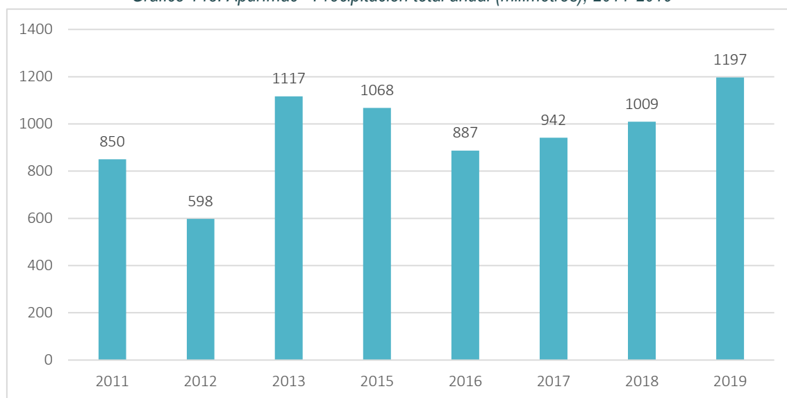
Gráfico 143: Apurímac - Precipitación total anual (milímetros), 2011-2019
