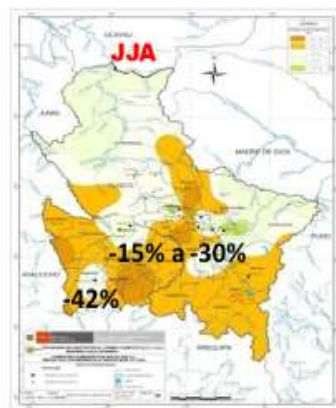
Mapa 28: Escenarios de cambio climático para Cusco y Apurímac al 2030
