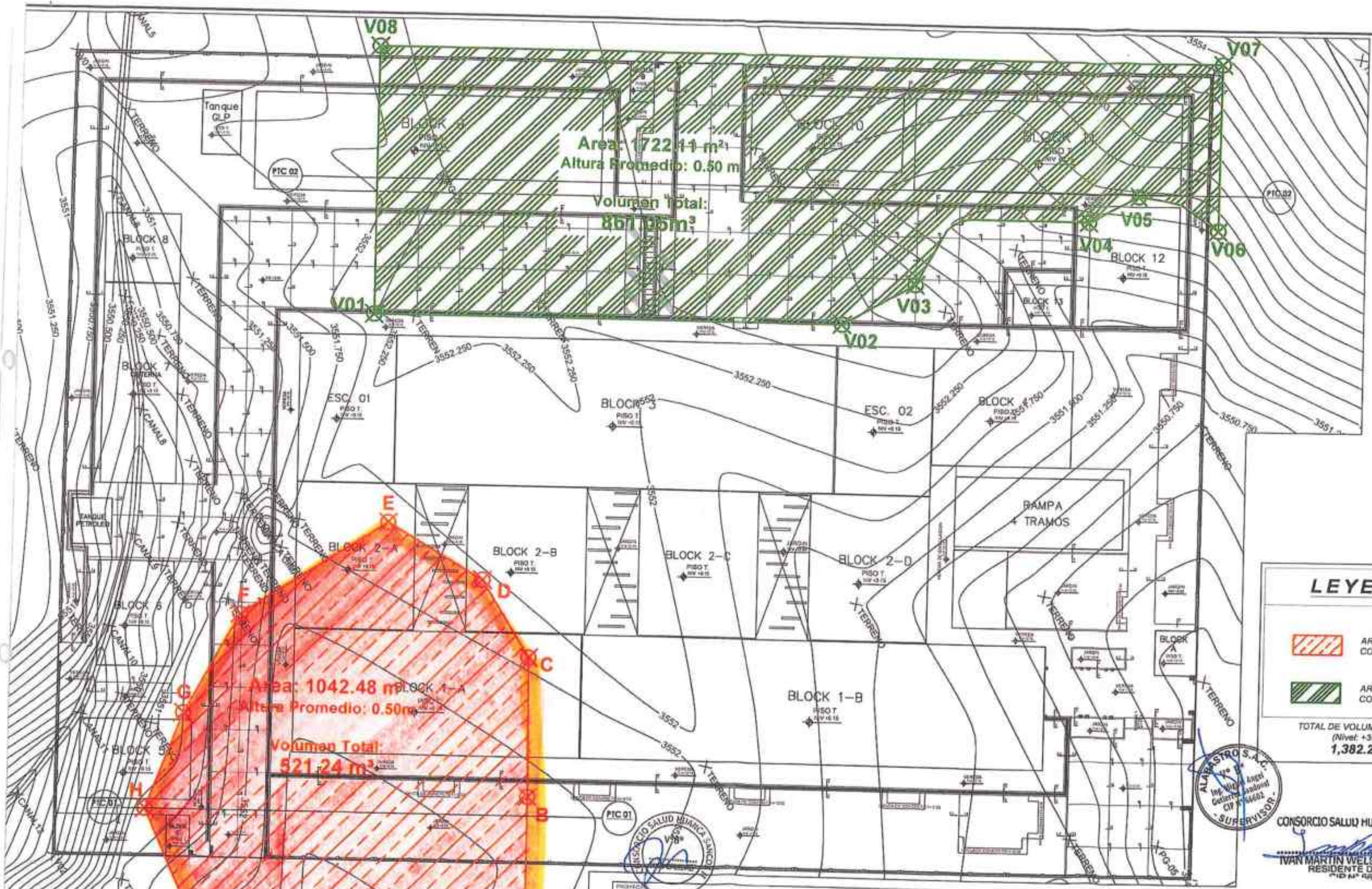
PLANTA DE MOVIMIENTO DE TIERRAS ESC: 1/350
