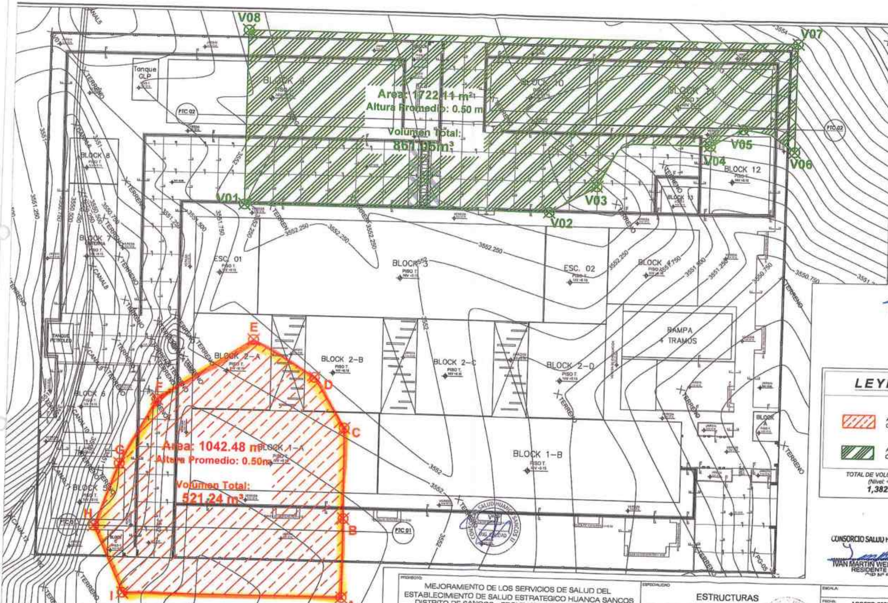
PLANTA DE MOVIMIENTO DE TIERRAS ESC: 1/350
