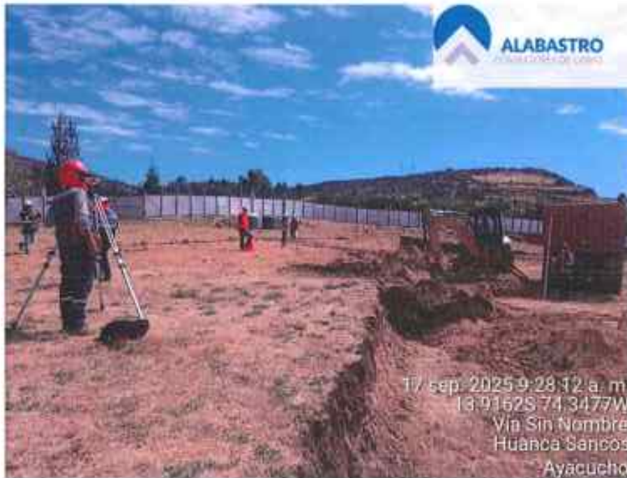
FOTO N°11: VERIFICACION DE EXCAVACION PARA ZAPATAS
