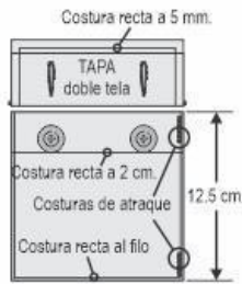
BOLSILLO DE MANGA detalle y medidas con la tapa abierta ( brazo derecho )
