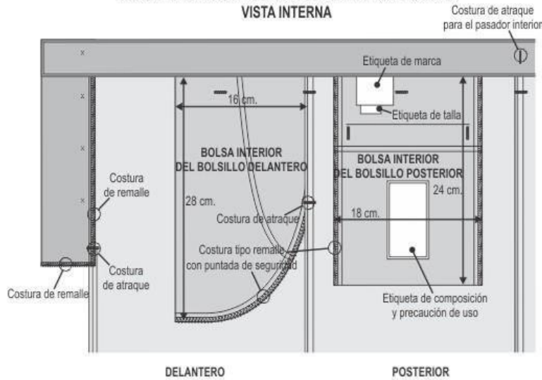
VISTA DE MEDIDAS Y DETALLE DE LA PRETINA Y JARETA VISTA INTERNA
