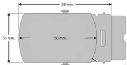
HEBILLA VISTA SUPERIOR
